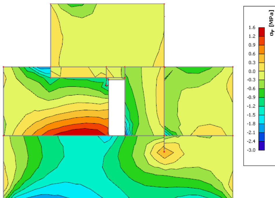
Slika 8.2.3 Tlačna naprezanja \sigma_y (Mpa) za nazovistalnu kombinaciju GSU
