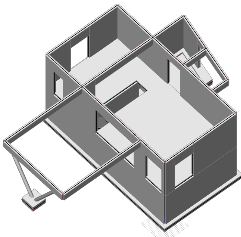
Slika 2.4 Proračunski model objekta – pogled
