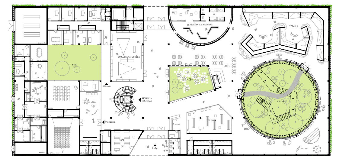
TLOCRT PRIZEMLJA
