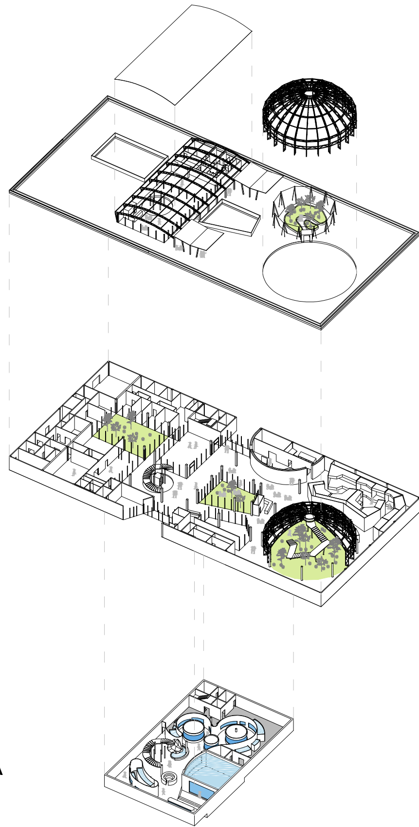
AKSONOMETRIJA
