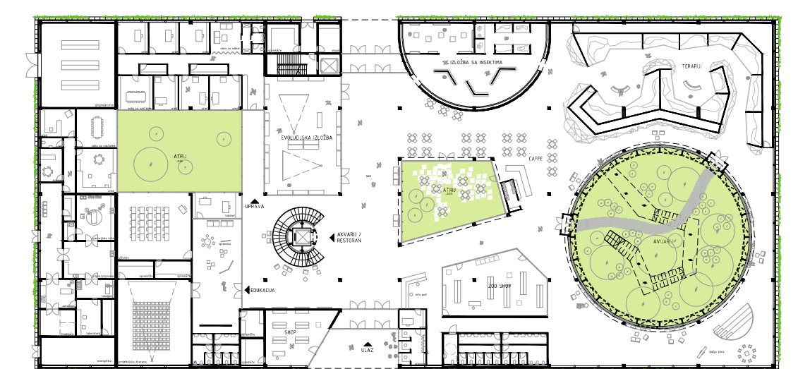
TLOCRT PRIZEMLJA
