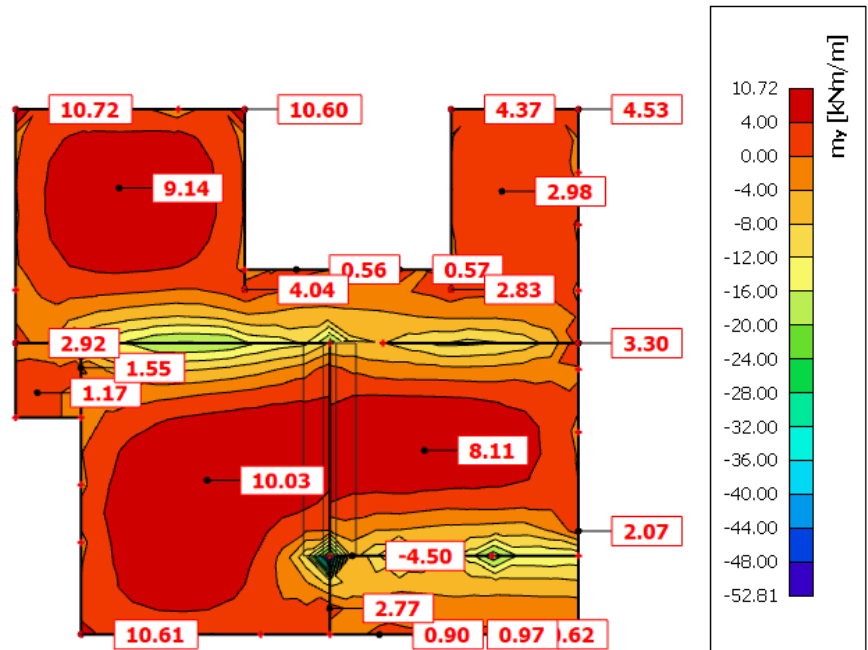
Moment m_y
