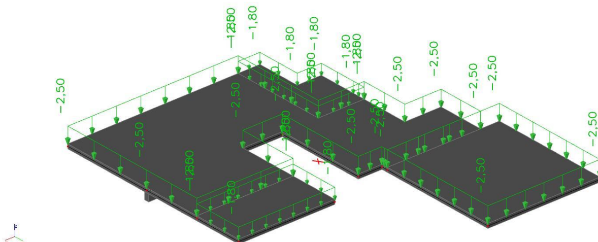
Slika 5.2.1 Dodatno stalno djelovanje G1 [ \text{kN/m}^2 ]
