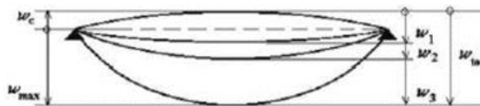
Slika 8.3 Prikaz progiba grede
