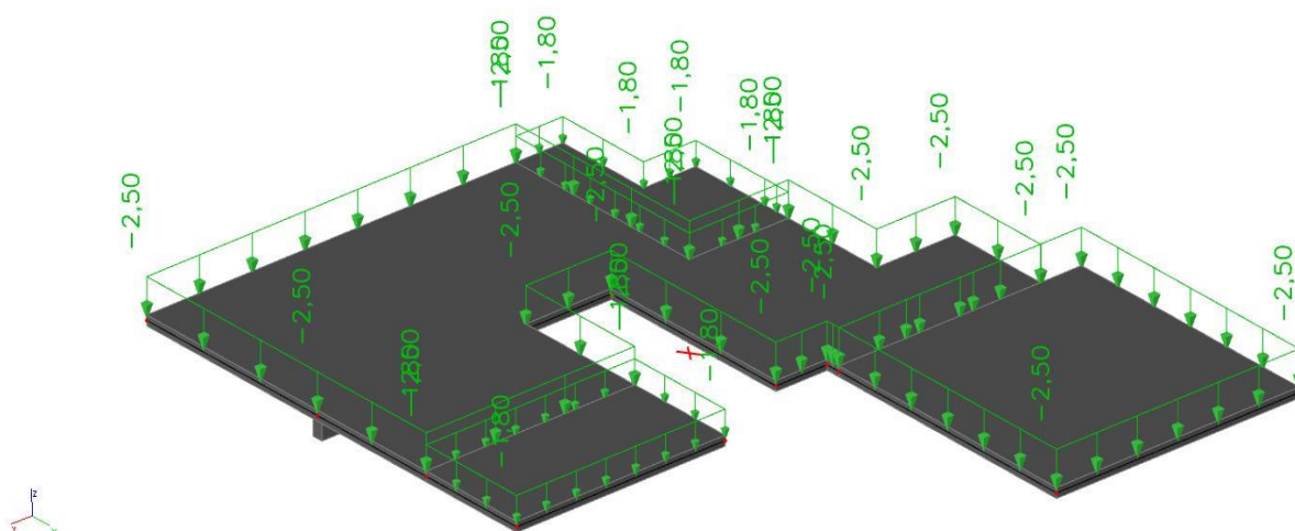
Slika 5.2.1 Dodatno stalno djelovanje G_1 [kN/m 2 ]
