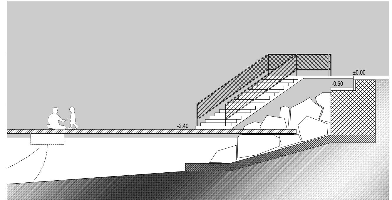
Presjek 1 M 1:100
