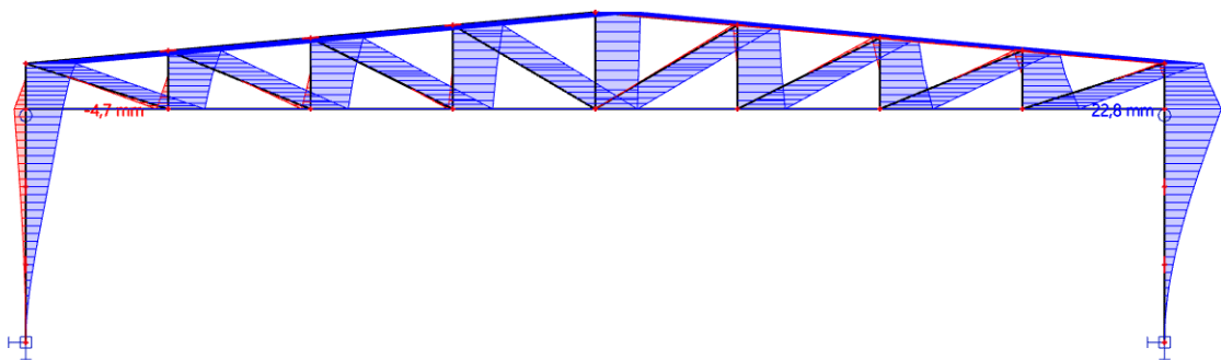
Slika 6 - Horizontalni progib glavnog nosača
