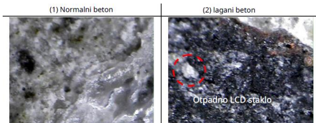
Slika 6. Zamjena od 5% otpadnim pijeskom LCD stakla [2]
