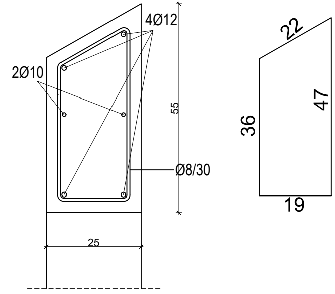
Presjek C-C
