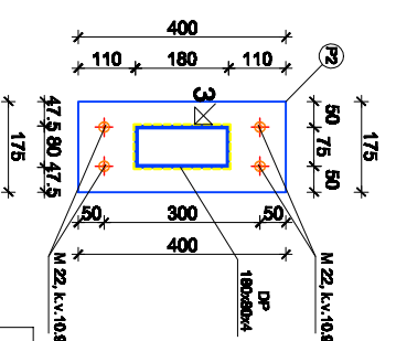
Presjek 2-2
