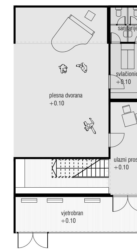
tlocrt prizemlja
