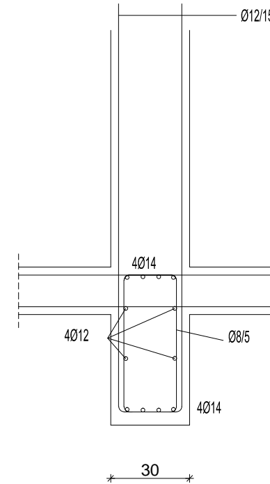
PRESJEK 2-2
