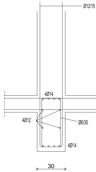
PRESJEK 1-1
