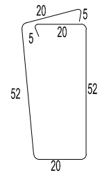
VILICE Ø6, Ø8 L=174 cm
