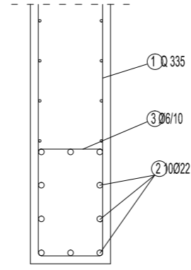
DETALJ "B"
