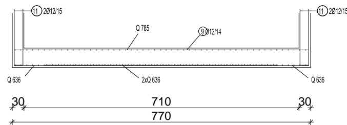
PRESJEK 1-1
