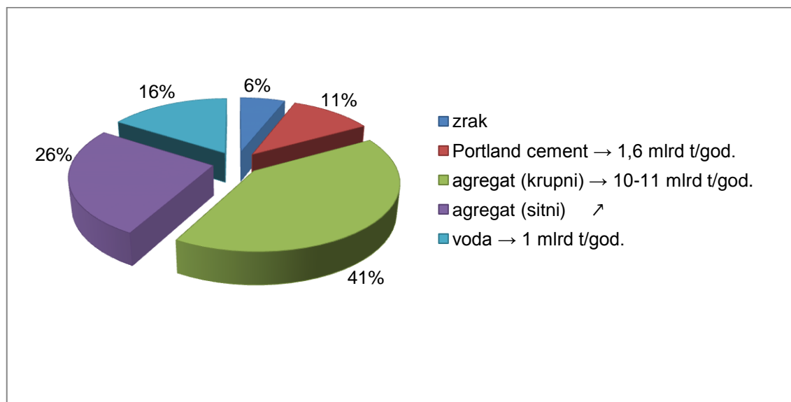
Slika 1.1 Volumni udio pojedinih sastojaka u betonu i njihova godišnja potrošnja u svijetu [7]
