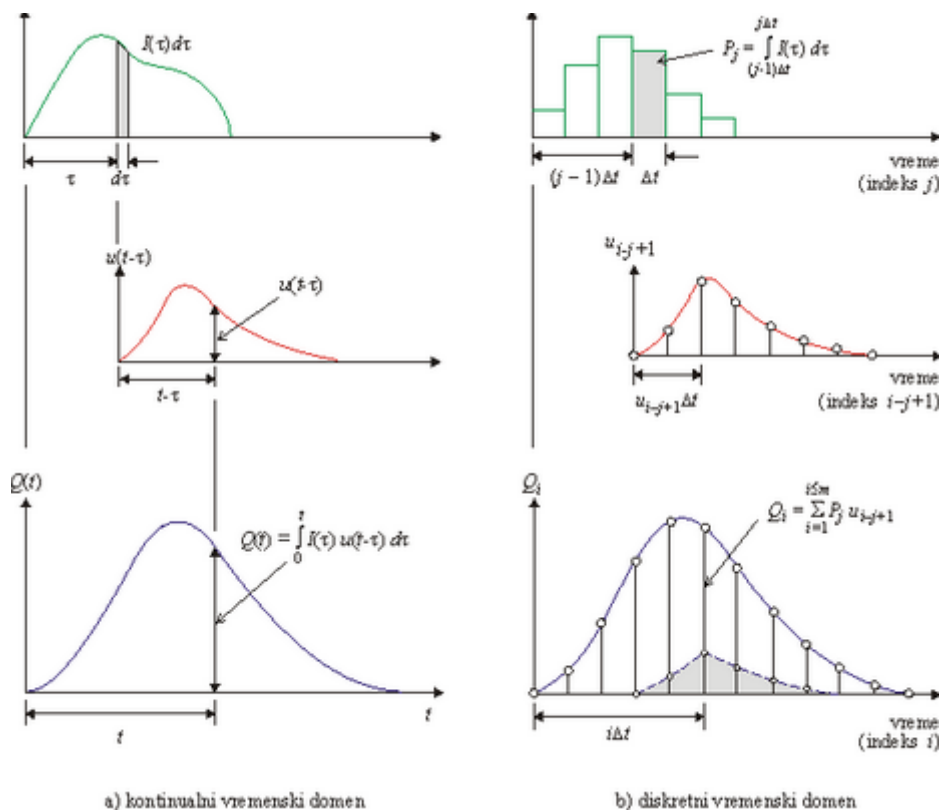
Slika 2.5. Shematski prikaz jediničnog hidrograma u kontinuiranom i diskretnom vremenu
