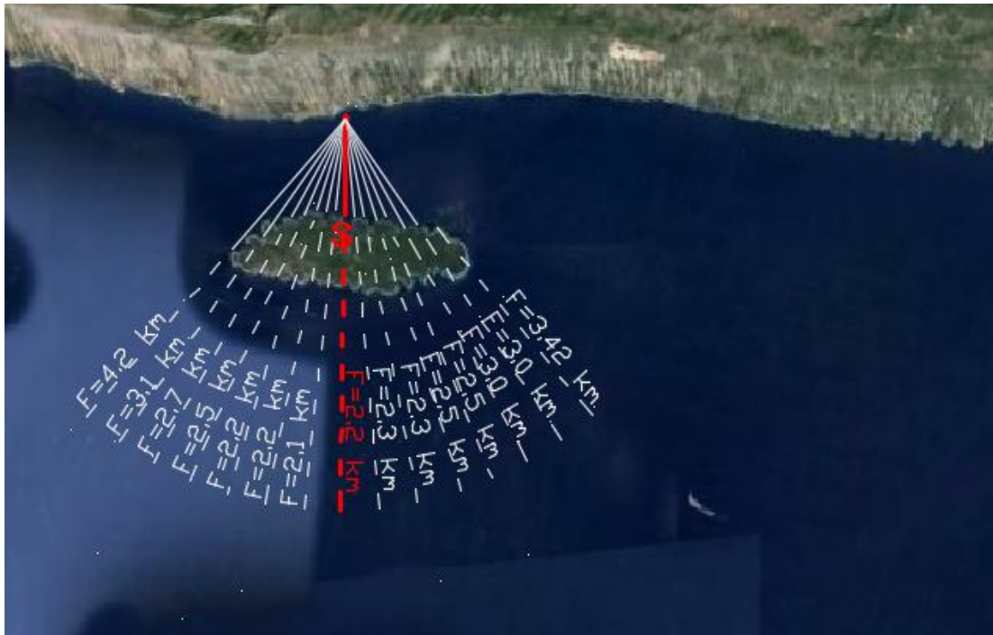
Slika 3.8. Skica za izračun efektivne duljine privjetrišta za centralni smjer S (80°)
