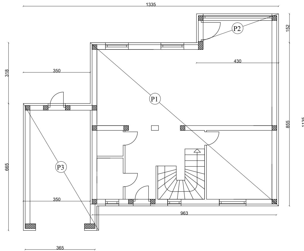
TLOCRT PRIZEMLJA
