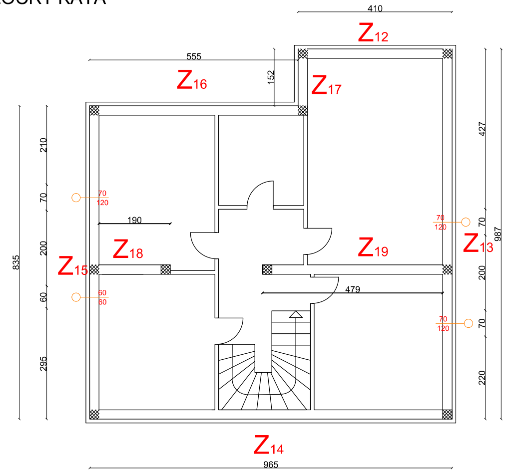
TLOCRT KATA
