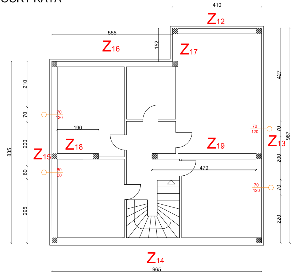
TLOCRT KATA
