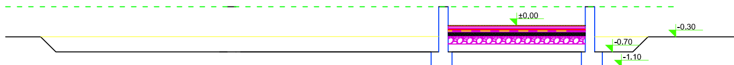
PRESJEK 2-2
