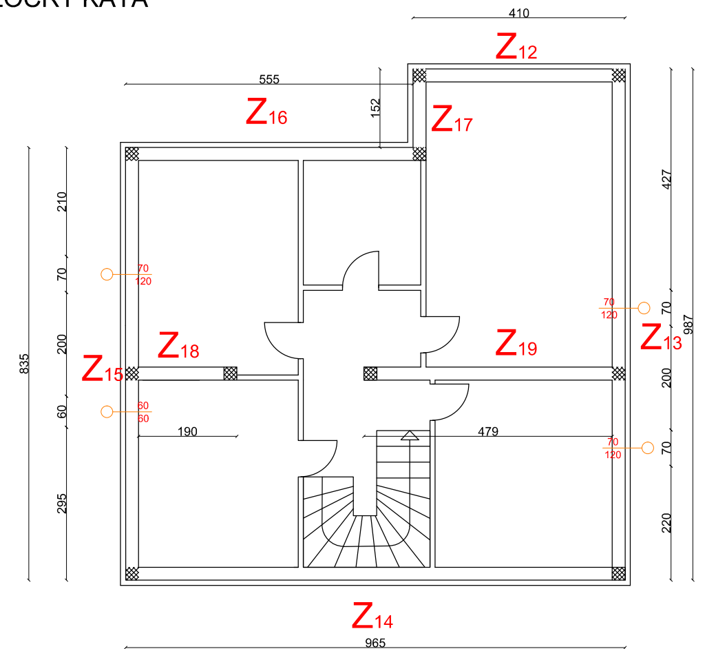
TLOCRT KATA
