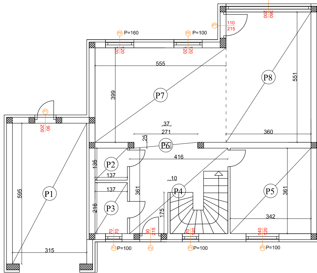
TLOCRT PRIZEMLJA
