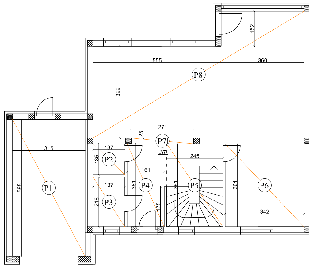
TLOCRT PRIZEMLJA
