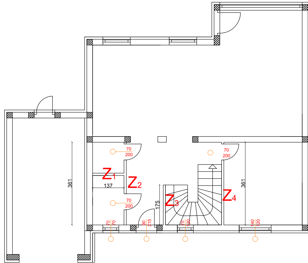
TLOCRT PRIZEMLJA
