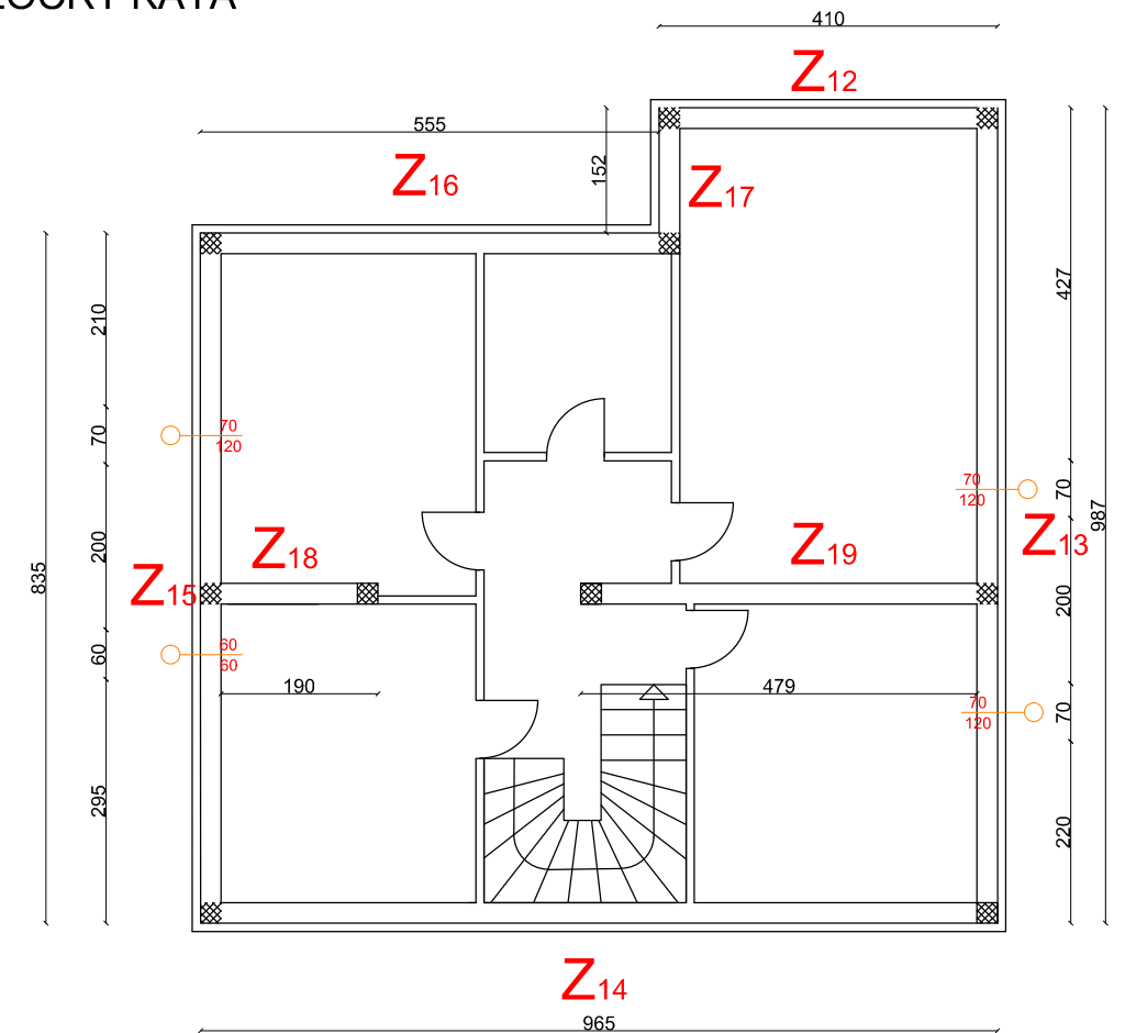
TLOCRT KATA
