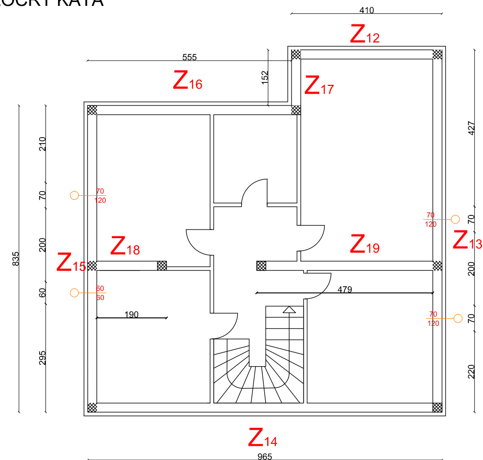
TLOCRT KATA
