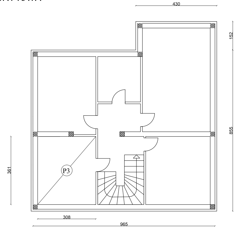
TLOCRT KATA
