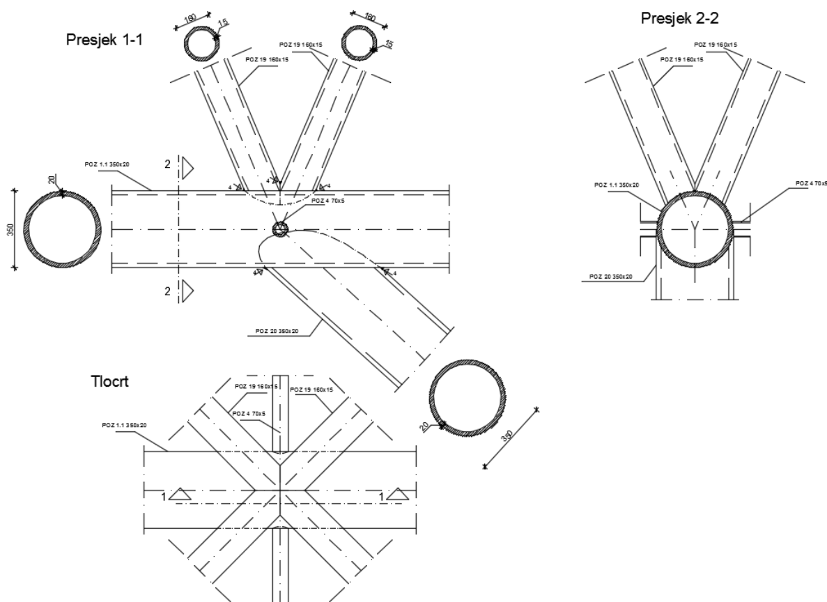
Slika 7.9. Montažni nastavak donjeg pojasa rešetke u smjeru x poviše stupa, Detalj M
