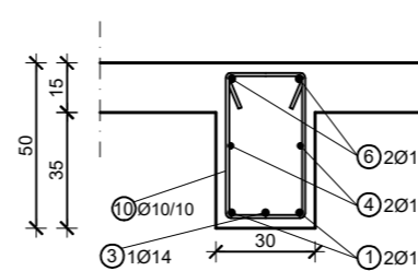
Presjek 4-4; MJ 1:25
