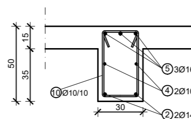
Presjek 3-3; MJ 1:25
