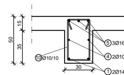
Presjek 1-1; MJ 1:25
