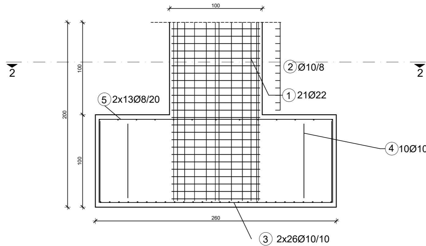
Presjek 3-3
