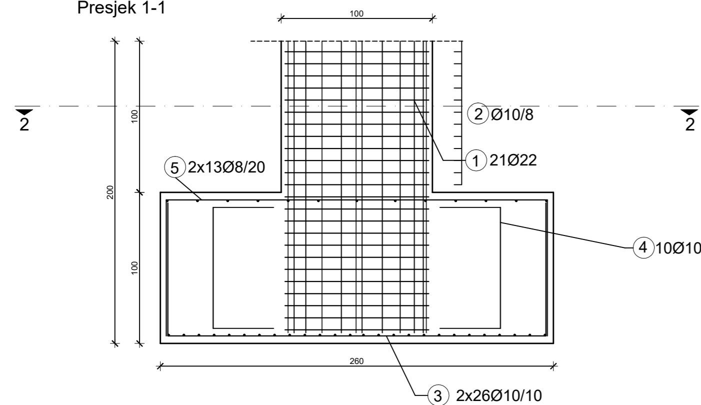
Presjek 1-1
