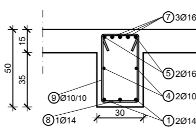
Presjek 3-3; MJ 1:25
