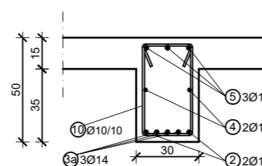
Presjek 3-3; MJ 1:25
