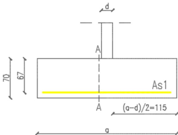
Slika12.2. Dimenzije trakastog temelja ispod zida debljine d=30\text{cm}
