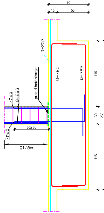
Presjek B-B
