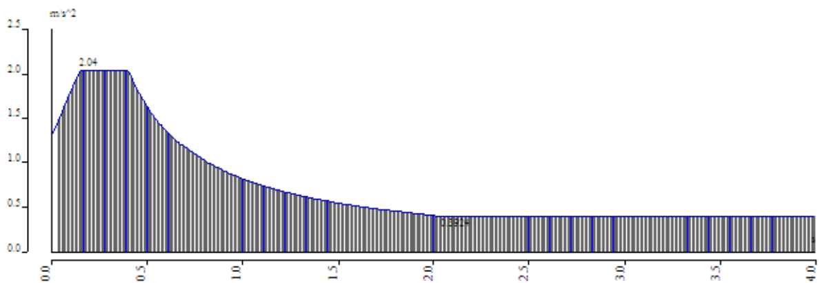
Slika 8.6 Normirani računski spektar odziva
