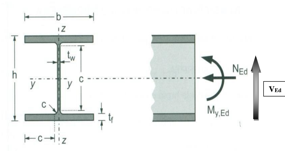
Slika 58 Poprečni presjek krovnog nosača
