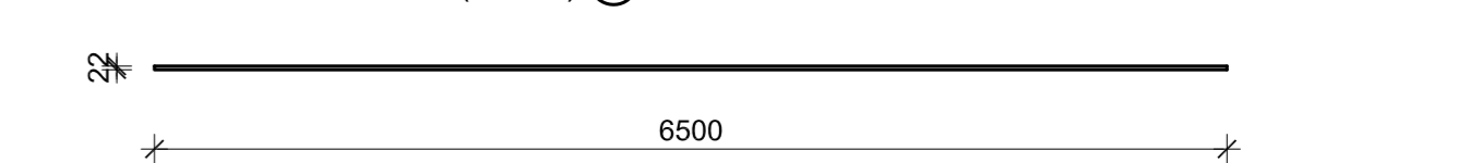
BOČNI SPREGOVI (SP2-1) Ø22, l=6500 mm, kom=16
