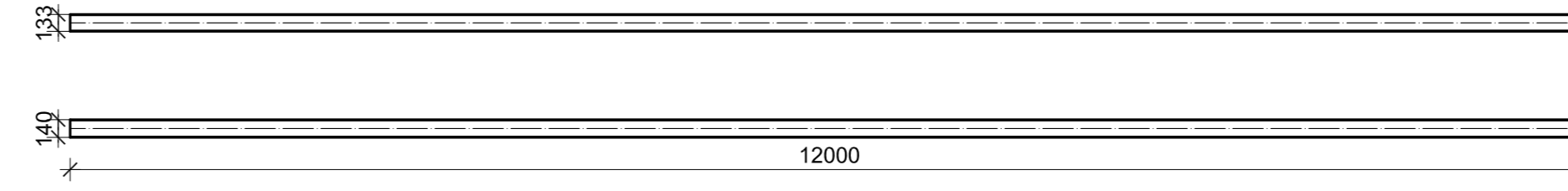
BOČNA PODROŽNICA (BP1-1) HEA 140, l=12000 mm, kom=18
