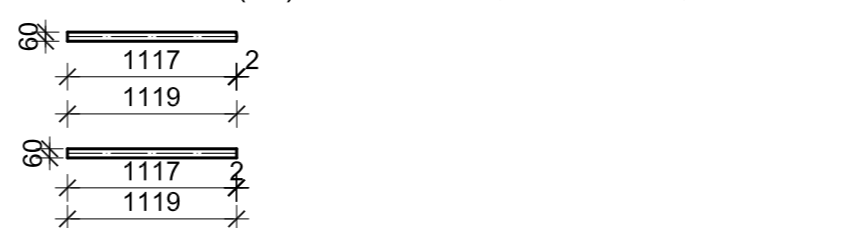
VERTIKALA (V5) 60X60X4, l=1119 mm, kom=1x11
