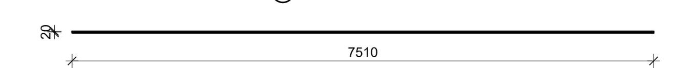
PROSTORNI SPREG Ø20, l=7510 mm, kom=4
