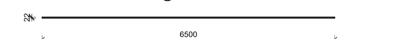
BOČNI SPREGOVI (SP2-1) Ø22, l=6500 mm, kom=16
