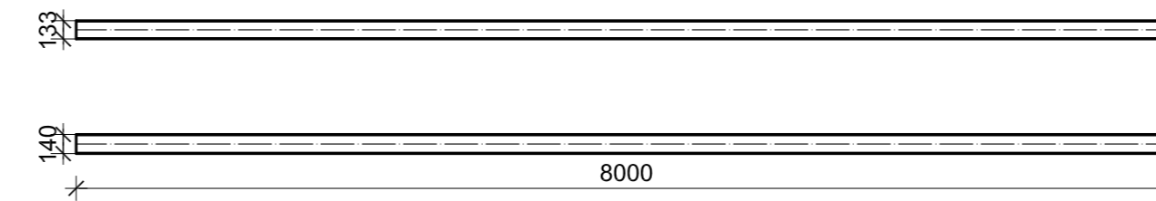
BOČNA PODROŽNICA (BP1-2) HEA 140, l=8000 mm, kom=18
