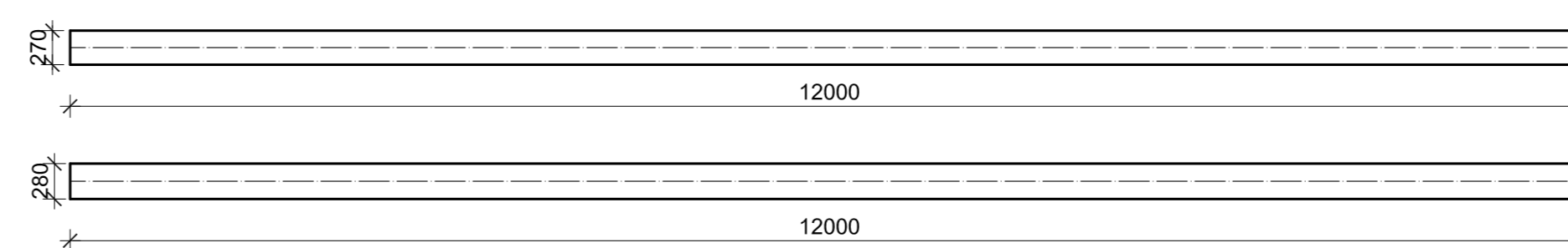
BOČNA PODROŽNICA (BP2-1) HEA 280, l=12000 mm, kom=6
