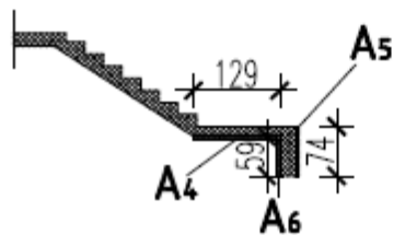
Presjek 2. podesta
