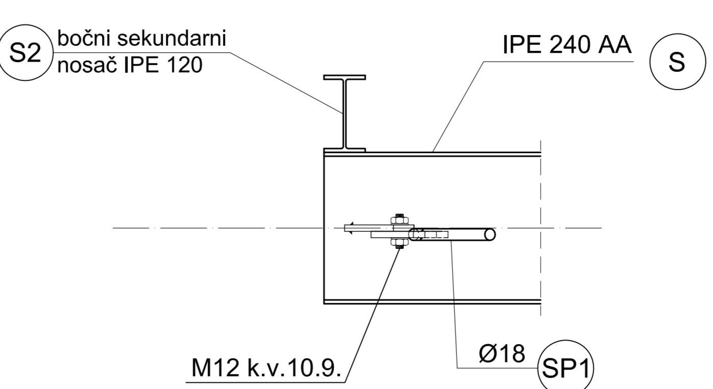
Presjek 2-2
