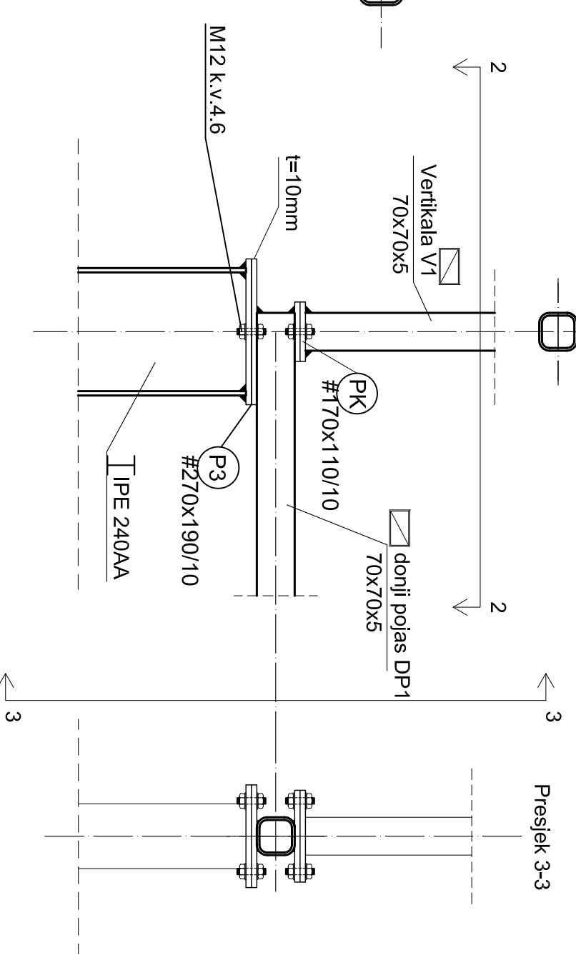
Presjek 2-2
