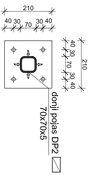
Presjek 1-1
