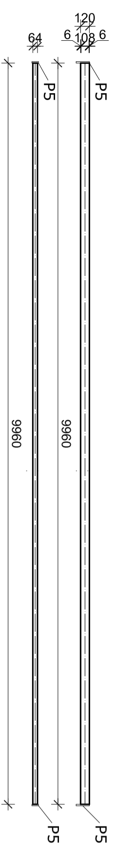
KROVNI SEKUNDARNI NOSAČI (S1-2) I IPE120, l=9960 mm, kom=20
