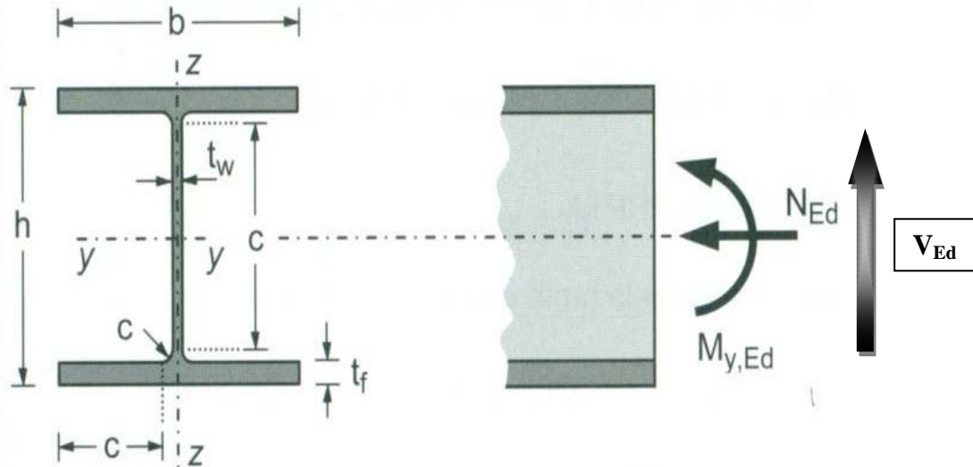
Slika 5.2.4.1 Poprečni presjek bočnih nosača
