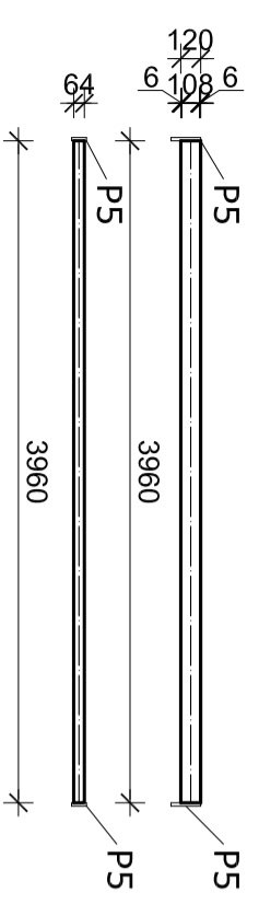
KROVNI SEKUNDARNI NOSAČI (S1-3) I IPE120, l=3960 mm, kom=10
