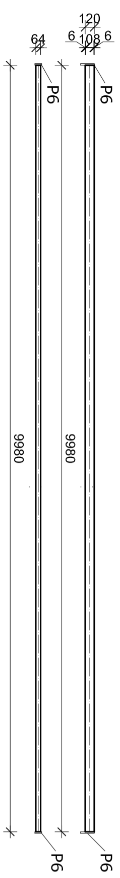
BOČNI SEKUNDARNI NOSAČI (S2-2) I IPE120, l=9980 mm, kom=16
