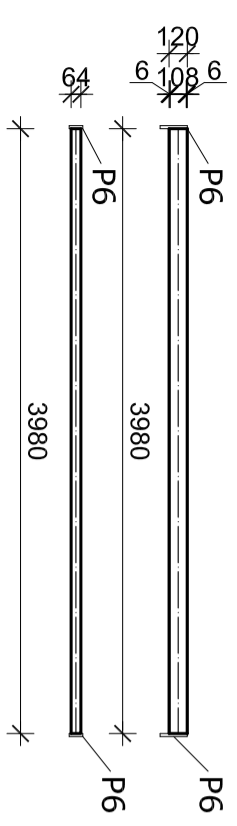
KROVNI SEKUNDARNI NOSAČI (S2-3) I IPE120, l=3980 mm, kom=8
