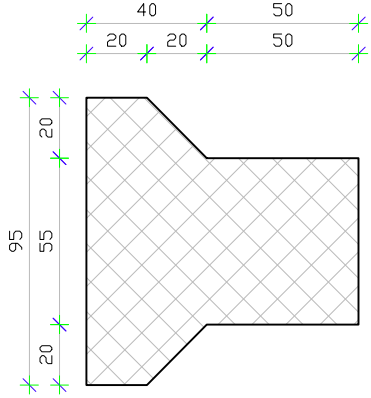
Presjek 1 - 1 M 1:25
