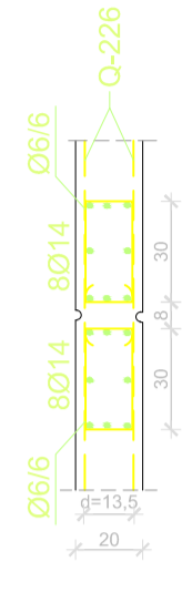
Zid u osi M - detalj F M 1:25
