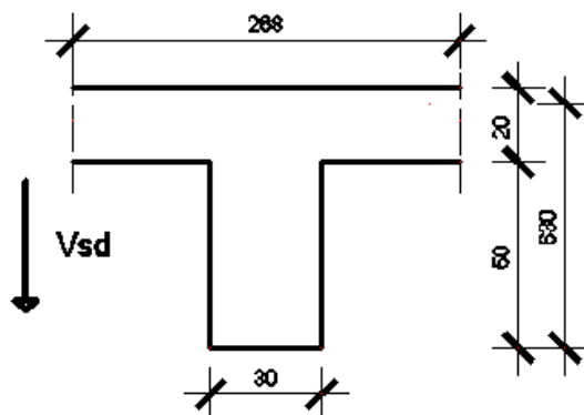
Slika 47: Poprečni presjek pozicije 106
