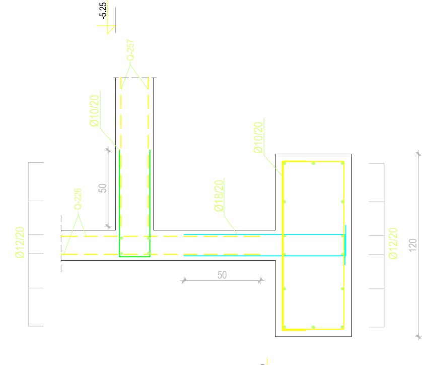
PRESJEK 4 - 4
