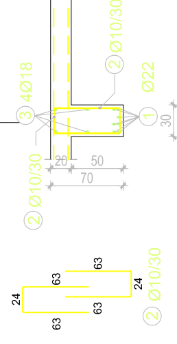
Detalj 1 M 1:50
