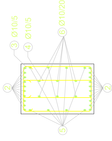
Presjek 2 - 2 M 1:25
