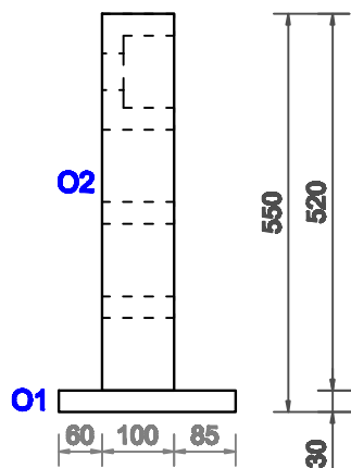
PRESJEK A-A
