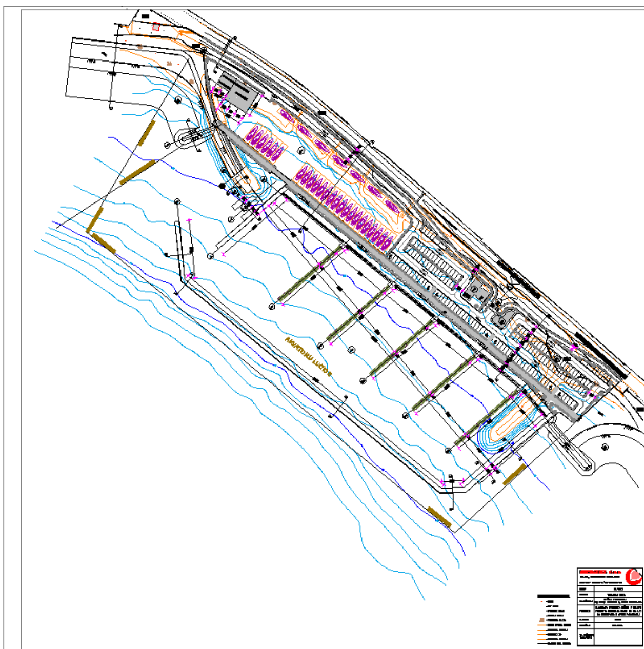
Slika 2. Situacija lučice
