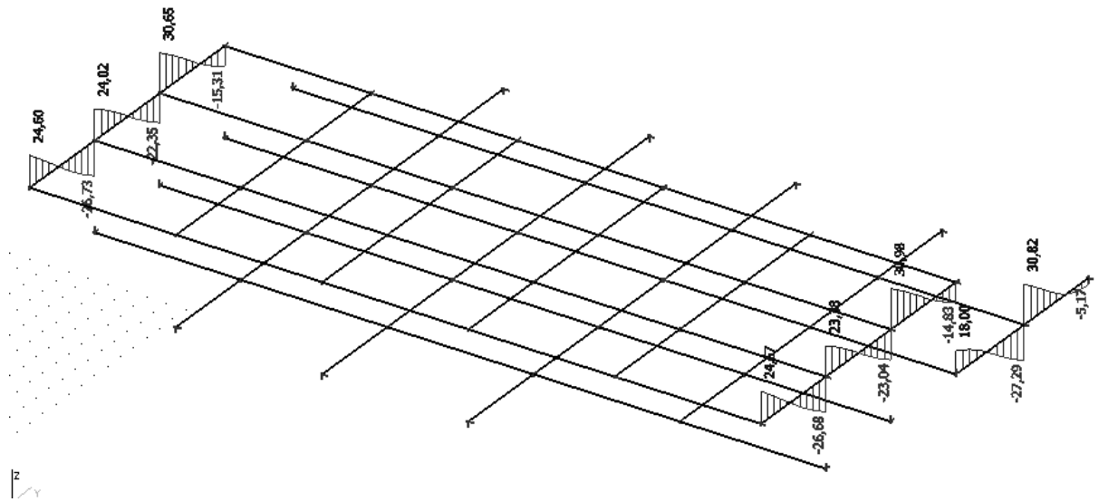
Slika 3.52. Dijagram poprečnih sila V_z (kN) za gredu G4 POZ 100 i 200 (vlastita težina i dodatno stalno opterećenje "dG")
