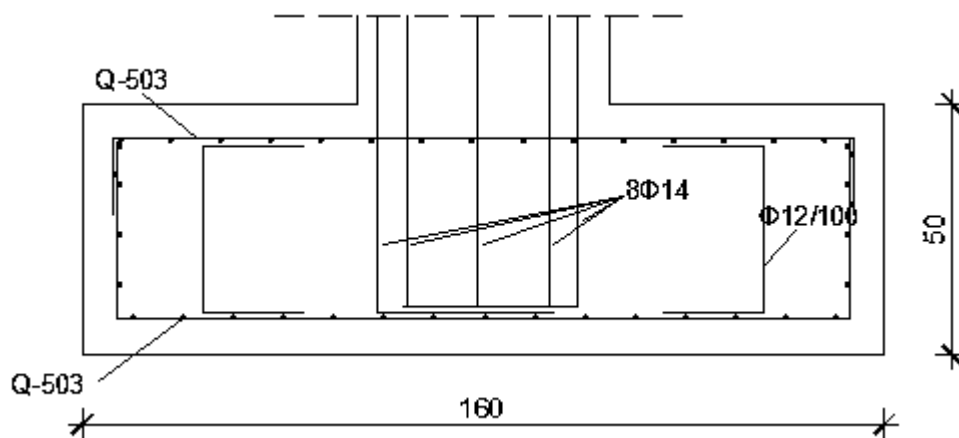
Slika 3.70. Skica armature temelja
