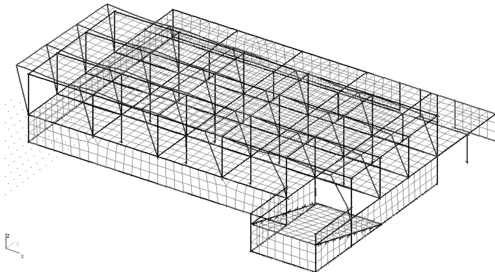
Slika 2.27. 1. oblik osciliranja: T=0,4518 s, S_x=31,79\%G_x , S_y=0,19\%G_y , S_z=0,0\%G_z
