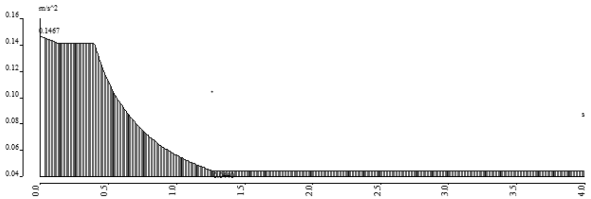
Slika 2.26. Računski spektar odziva
