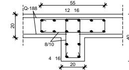
Detalj K
