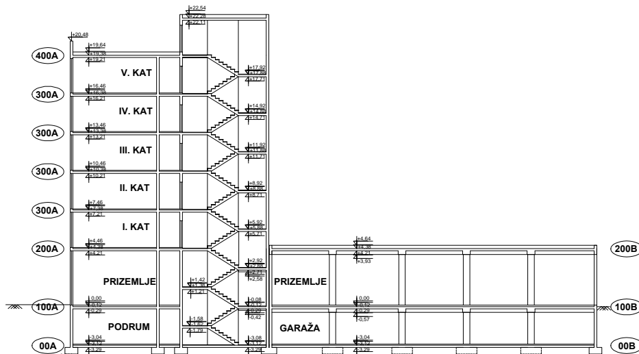
PRESJEK B-B
