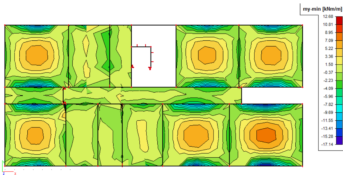
Slika 3.7. Dijagram momenata savijanja M_y (vlastita težina i dodatno stalno opterećenje „dG“)
