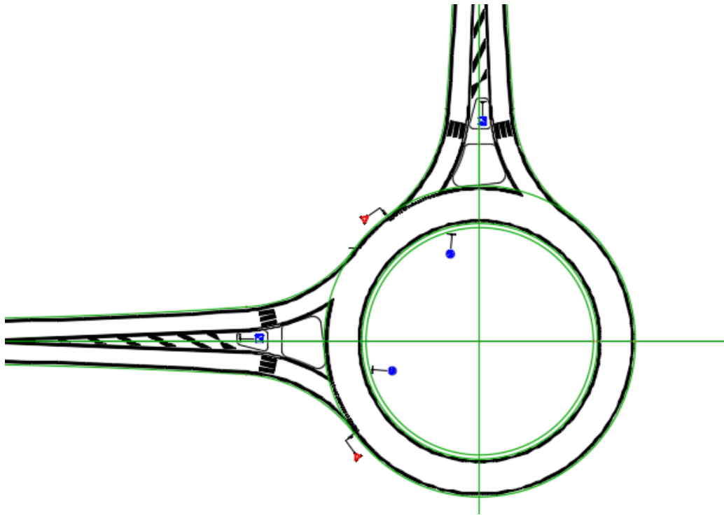
Slika 5.13. Tlocrtni prikaz jednostračnog kružnog raskrižja [9]
