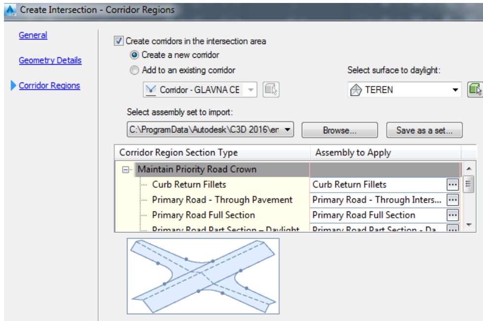
Slika 4.15. Defininiranje regija koridora [9]
