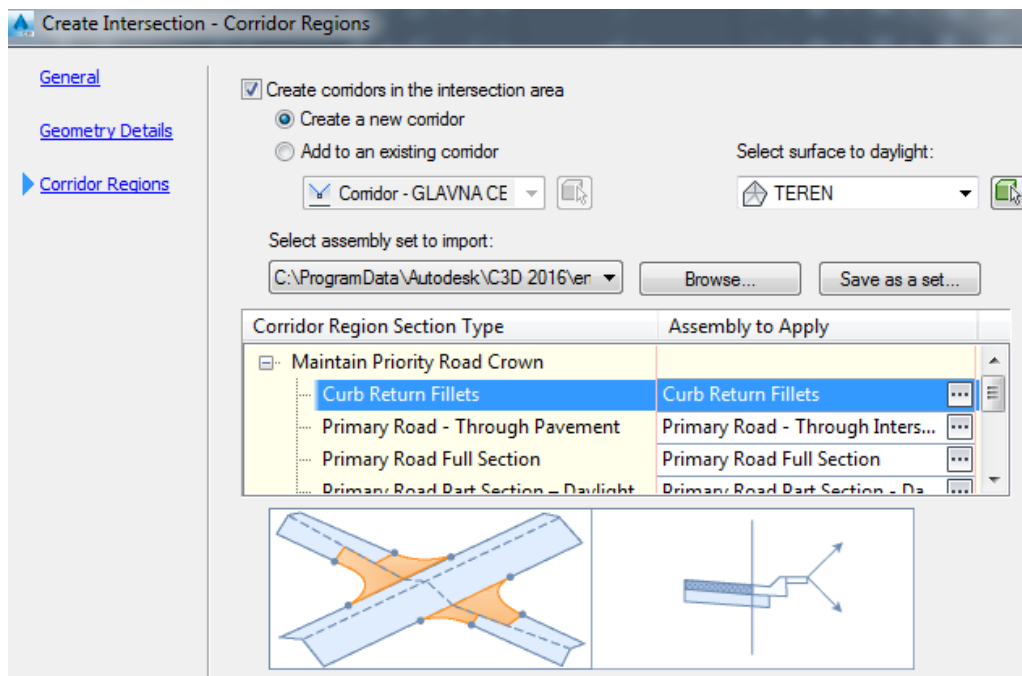
Slika 4.16. Defininiranje regija koridora – rub kolnika [9]
