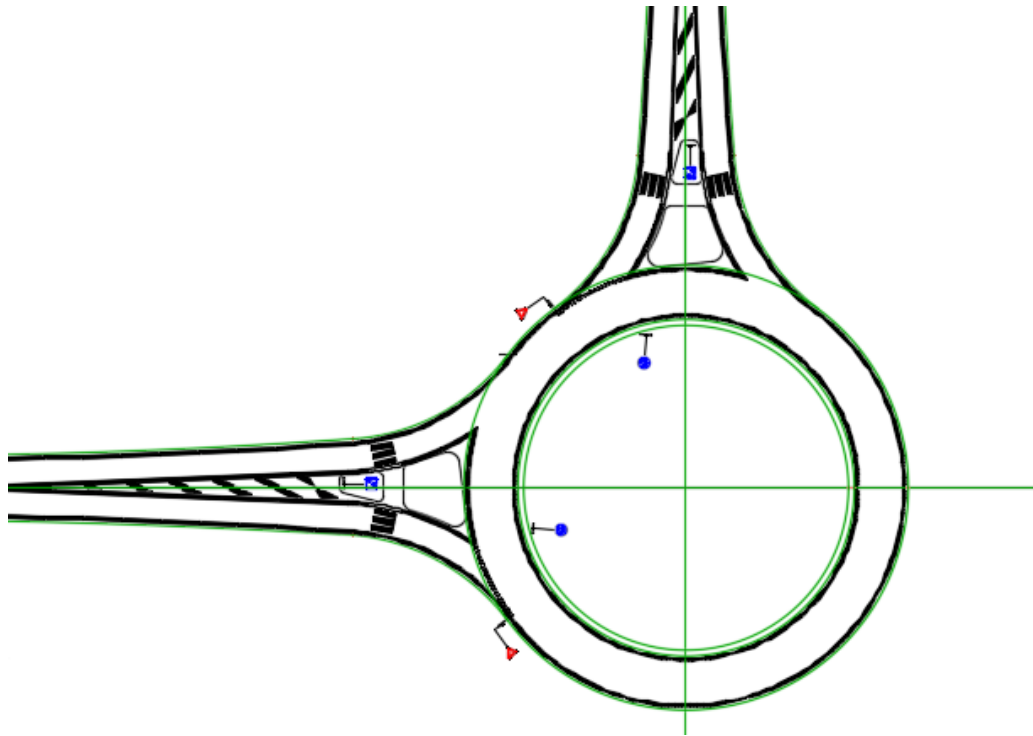
Slika 5.13. Tlocrtni prikaz jednotračnog kružnog raskrižja [9]
