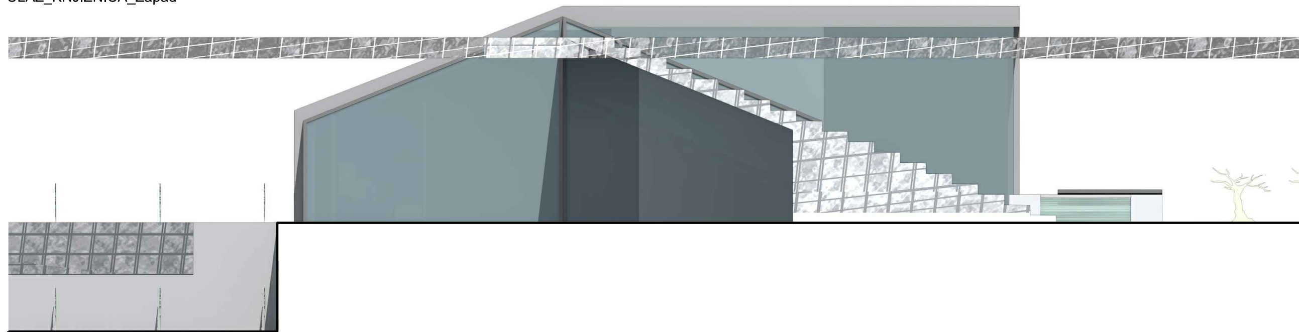
PROČELJE_STAKLENIK_Jug
