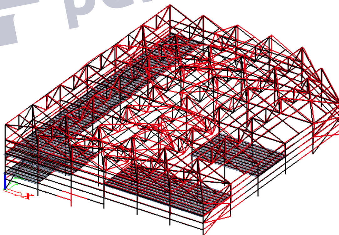
Slika 72: Prikaz deformacije konstrukcije
