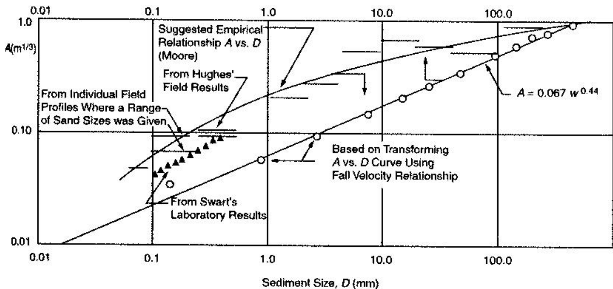
Slika 6.2. Dean-ov dijagram
