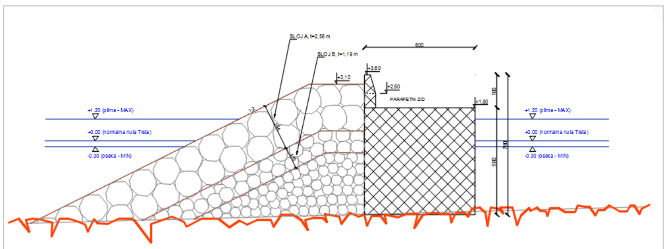
Slika 7.8. Poprečni presjek lukobrana
