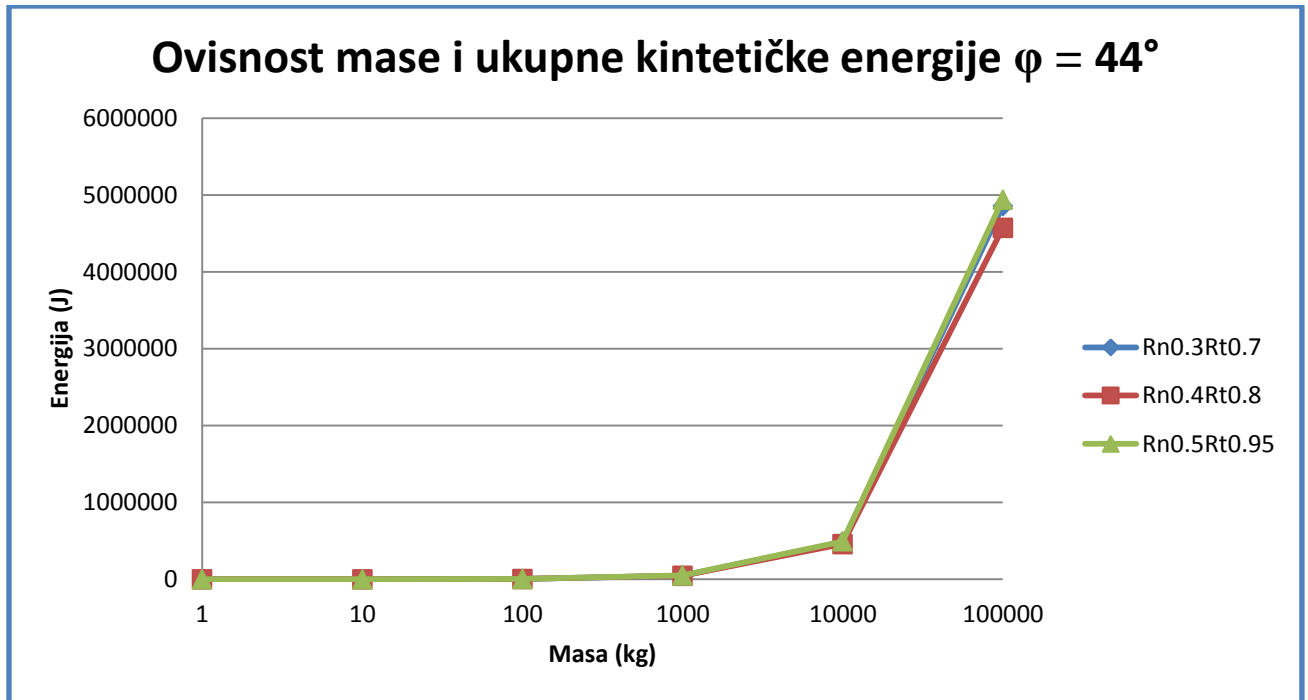
Dijagram 3. Ovisnost mase i energije prije sudara za kut trenja 44^\circ
