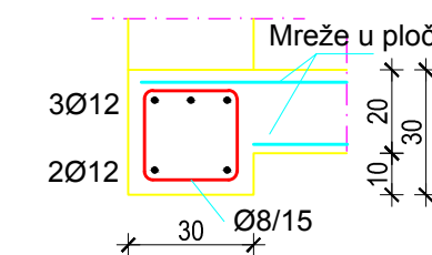
Presjek D-D:
