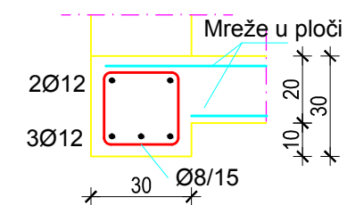
Presjek C-C:
