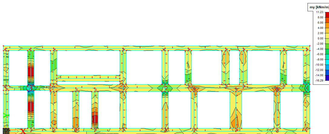
Crtež 8.40. Potrebna armatura [ \text{cm}^2/\text{m} ] u Y smjeru
