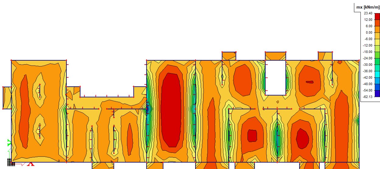
Crtež 8.4. Prikaz momenata savijanja m_x [kNm/m] na pločama za osnovnu kombinaciju GSN-1: 1,35*(G_0+G) + 1,5Q
