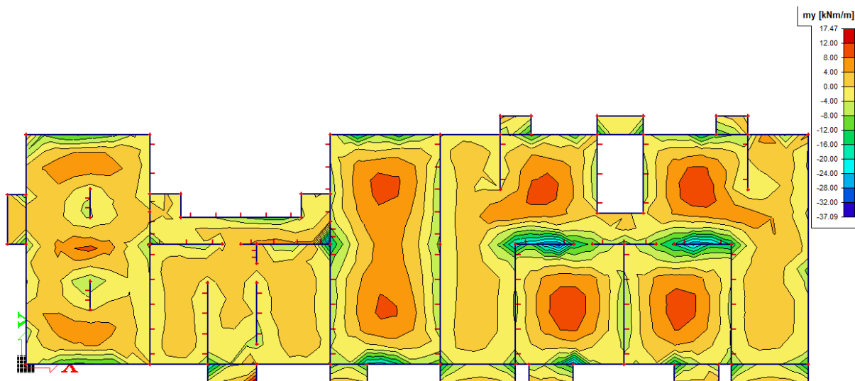
Crtež 8.5. Prikaz momenata savijanja m_y [kNm/m] na pločama za osnovnu kombinaciju GSN-1: 1,35*(G_0+G) + 1,5Q
