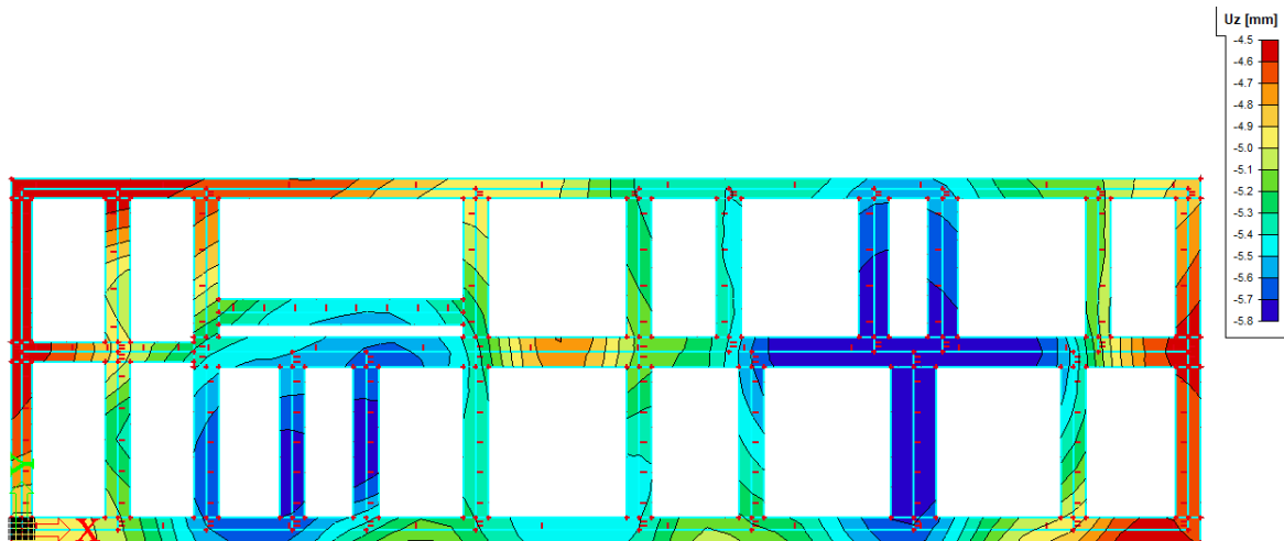
Crtež 8.36. Slijeganje temeljnih stopa U_z [mm] za kombinaciju GSU-1: 1,0*(G_0+G) + 0,5Q
