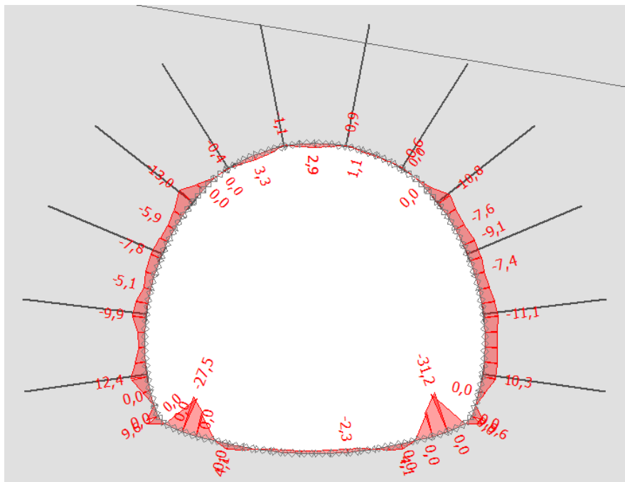
Slika 83. Momenti primarne podgrade za vertikalni iskop (kNm/m)
