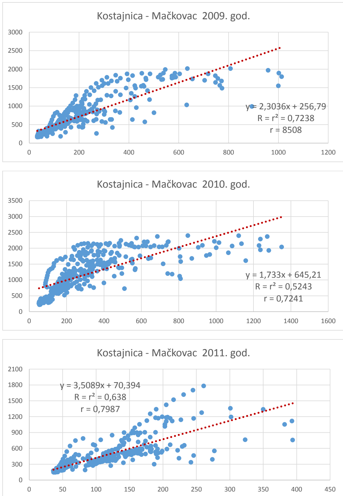
Slika 7.5.: Korelacija srednjih dnevnih protoka za mjerne stanice Kostajnicu i Mačkovac za 2009.-2011. god.
