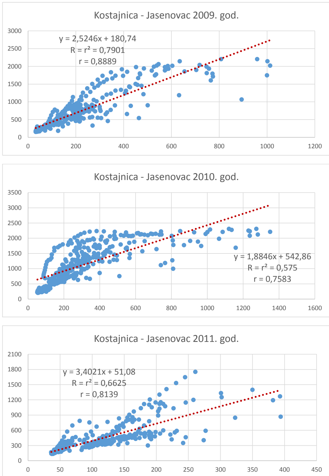
Slika 7.4.: Korelacija srednjih dnevnih protoka za mjerne stanice Kostajnicu i Jasenovac za 2009.-2011. god.
