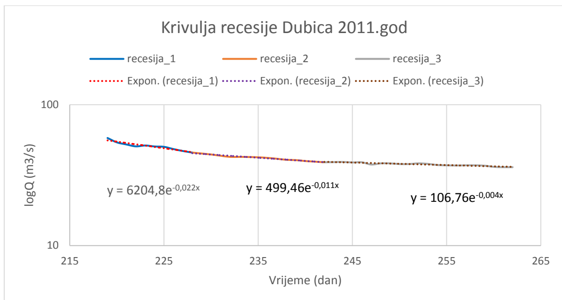
Slika 6.26.: Krivulje recesije – Dubica – 11.06.-16.10.2011. god.
