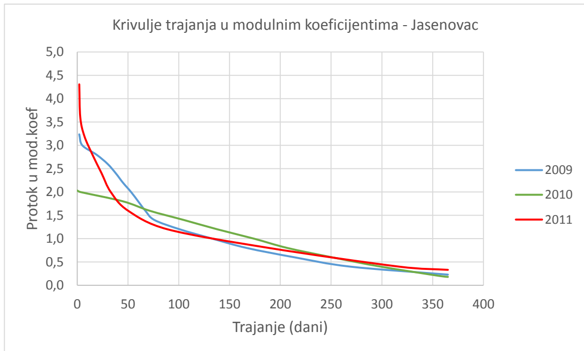
Slika 5.18.: Krivulje trajanja protoka u modulnim koeficijentima – Jasenovac – 2009.–2011. god.
