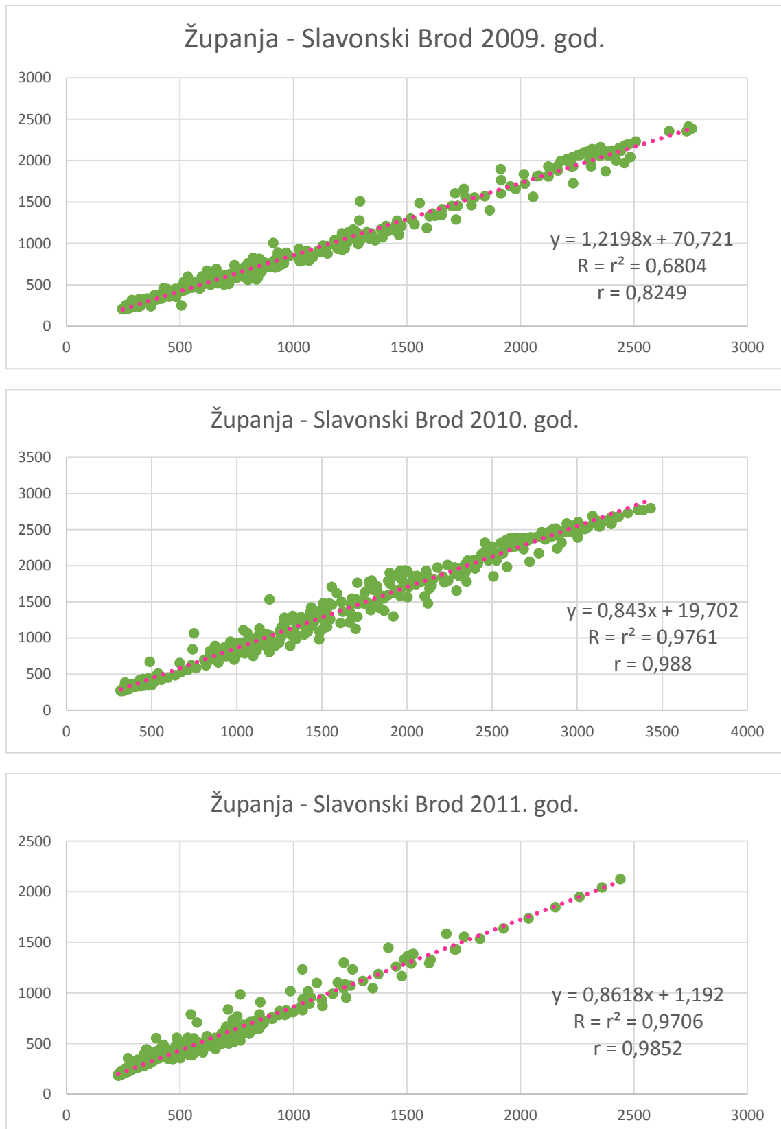
Slika 7.9.: Korelacija srednjih dnevnih protoka za mjerne stanice Županju i Slavonski Brod za 2009.-2011. god.
