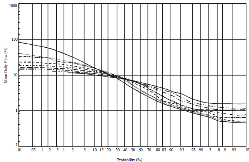
Slika 5.24.: Krivulja trajanja protoka za rijeku Ballinderry, tipična za kvalitetno snimljene podatke
