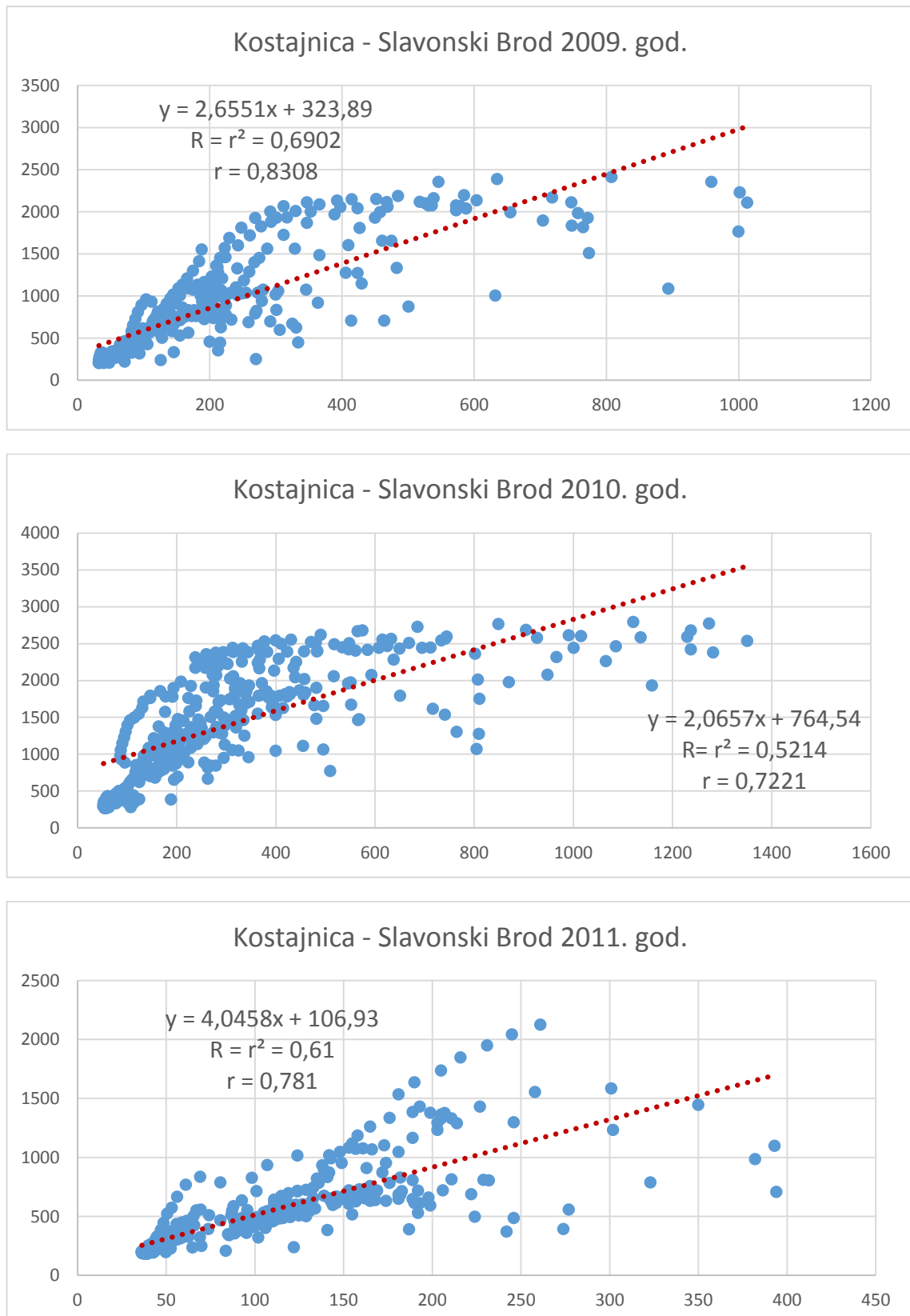
Slika 7.6.: Korelacija srednjih dnevnih protoka za mjerne stanice Kostajnicu i Slavonski Brod za 2009.-2011. god.
