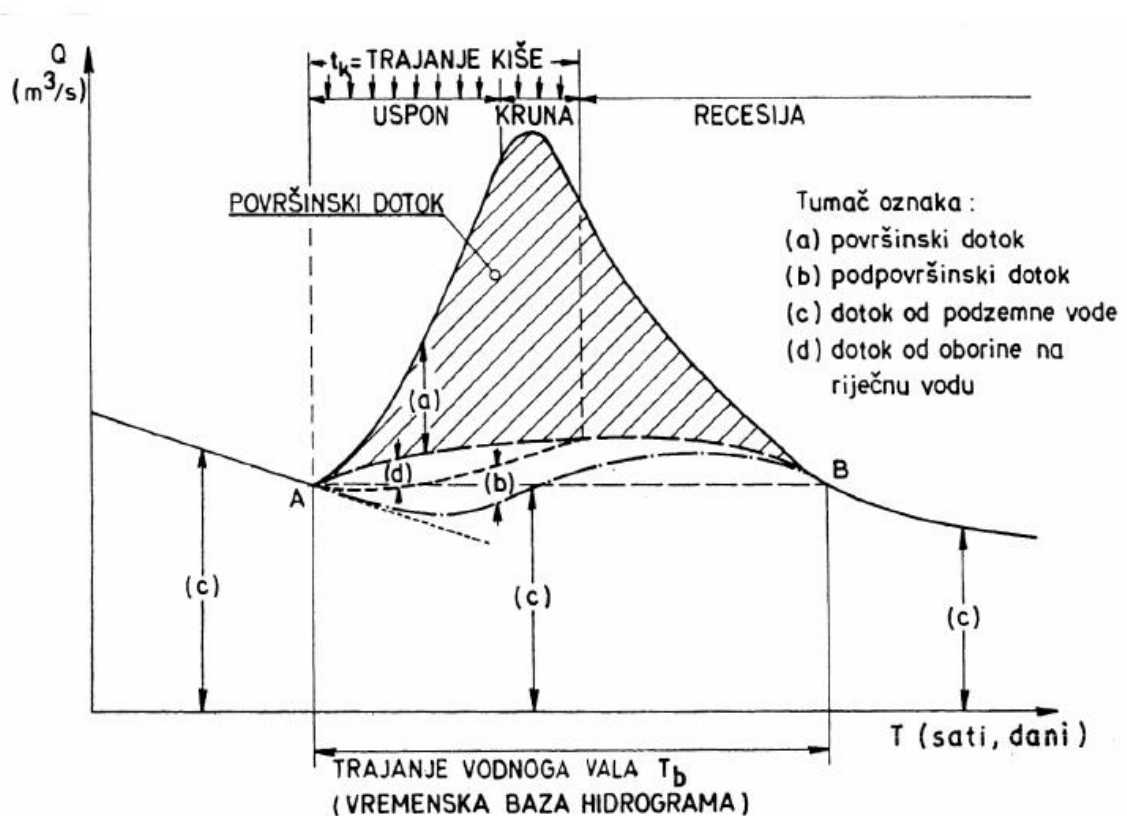
Slika 4.4. : Glavni dijelovi hidrograma otjecanja
