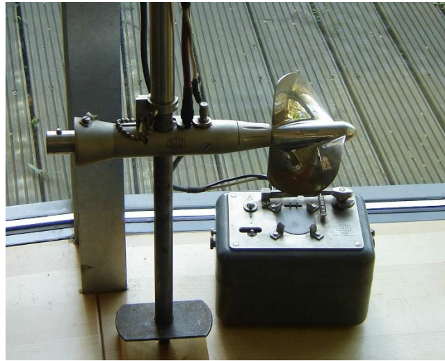
Slika 4.2.: Hidrometrijsko krilo
