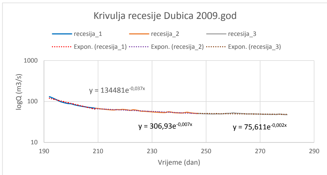
Slika 6.25.: Krivulje recesije –Dubica – 04.06.-07.10.2009. god.
