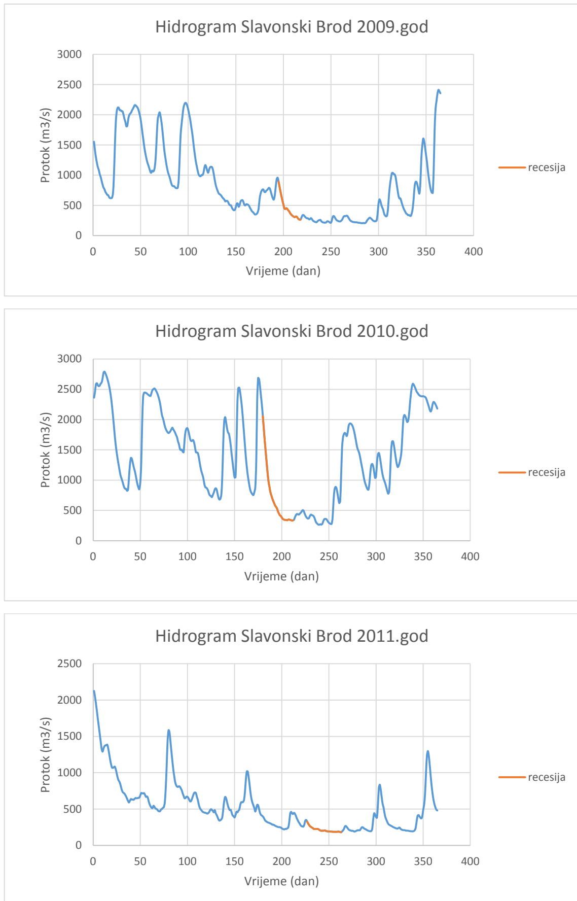
Slika 4.9.: Hidrogrami za mjernu stanicu Slavonki brod za 2009. – 2011. godinu
