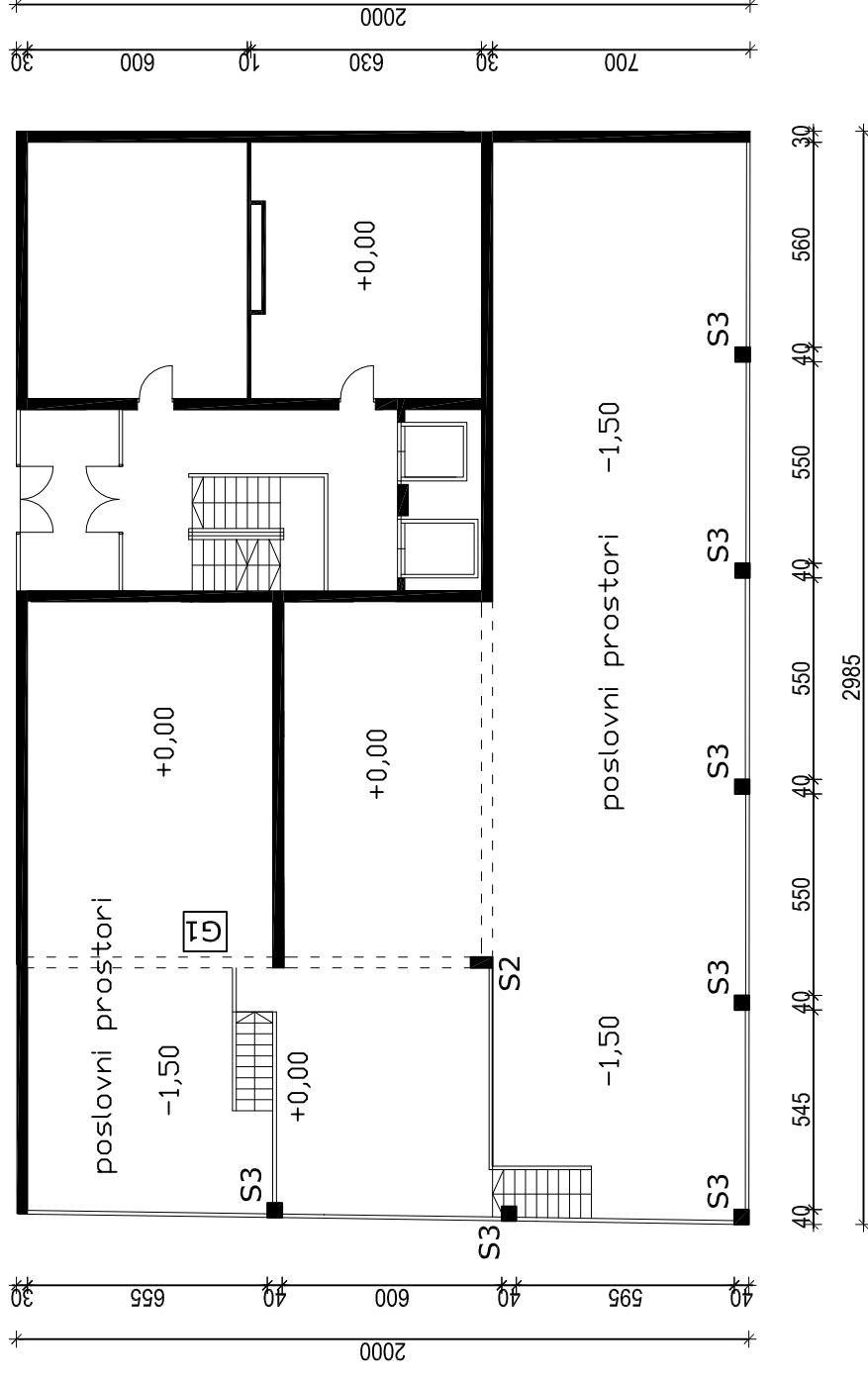
Prizemlje južnog tornja
