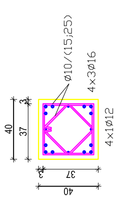
PRESJEK A-A
