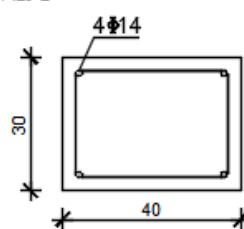
DETALJ 2
