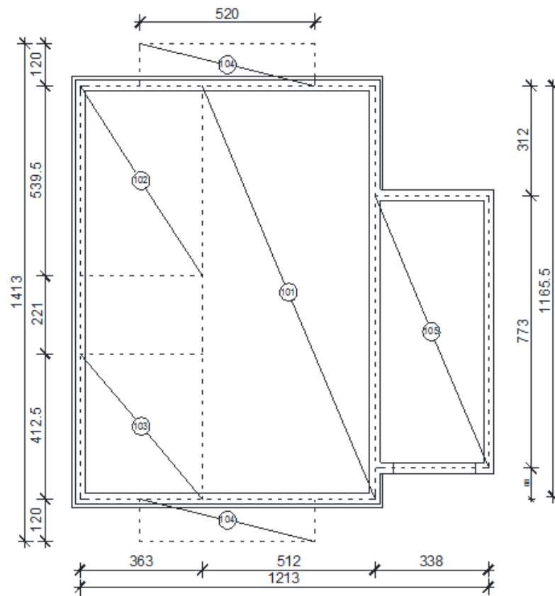
Slika 10.1. Prikaz pozicija 1. kata
