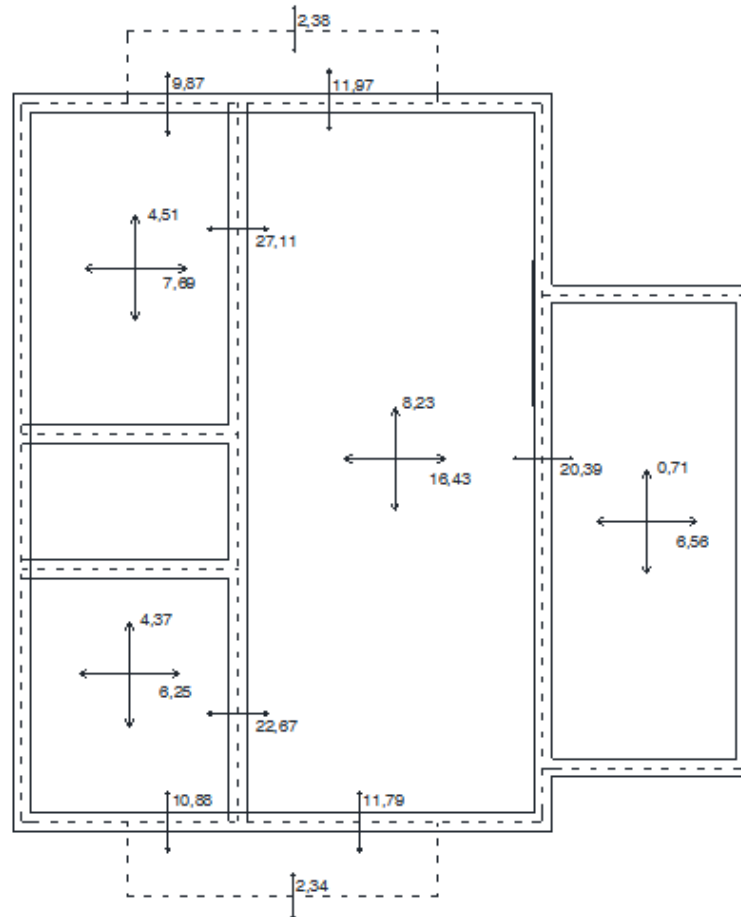
Slika 10.2.1. Prikaz maksimalnih momenata u poljima i na ležajevima
