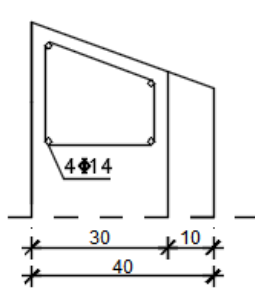
presjek 1-1
