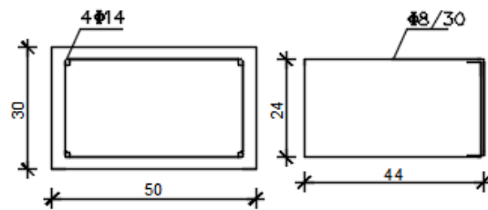
DETALJ 5
