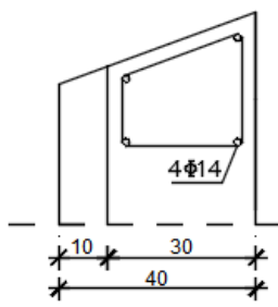
presjek 2-2
