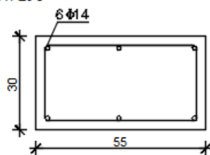
DETALJ 3
