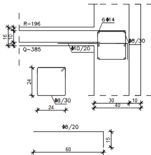
presjek 1-1
