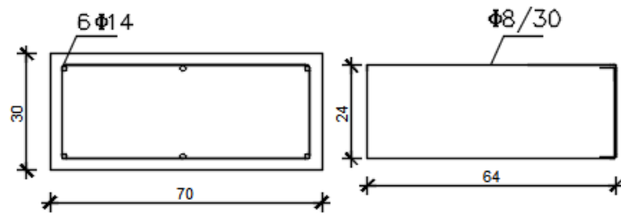
DETALJ 4
