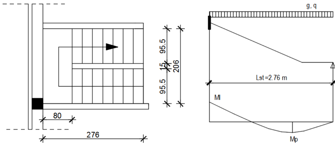
Slika 11.1.1 Tlocrt stubišta
