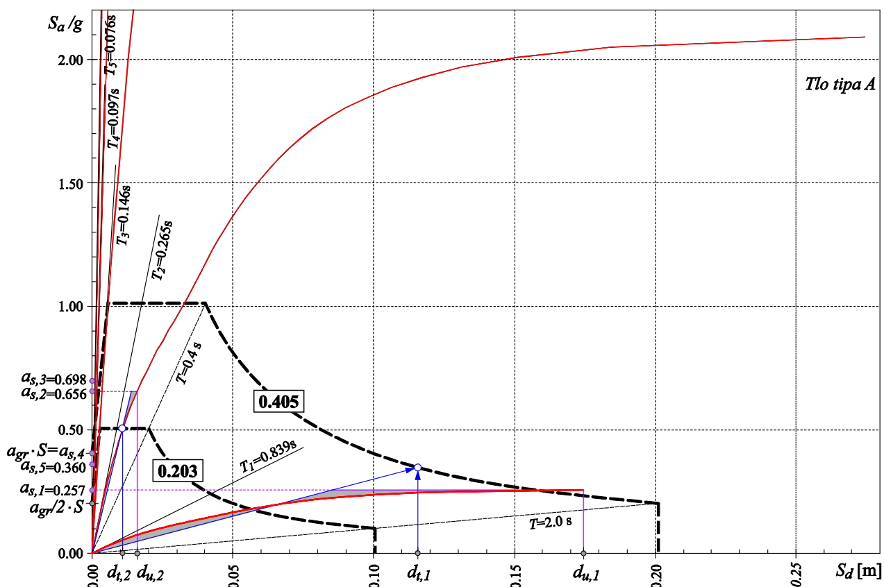
Crtež 2.12 Određivanje spektralnog ubrzanja modova, 5-katnog a/b okvira u x smjeru, uz elastični spektralni odgovor tla za ubrzanje tla 0.405g ( a_{s,1} ) i 0.203g ( a_{s,2} - a_{s,5} ), (SRSS kombinacija modova)
