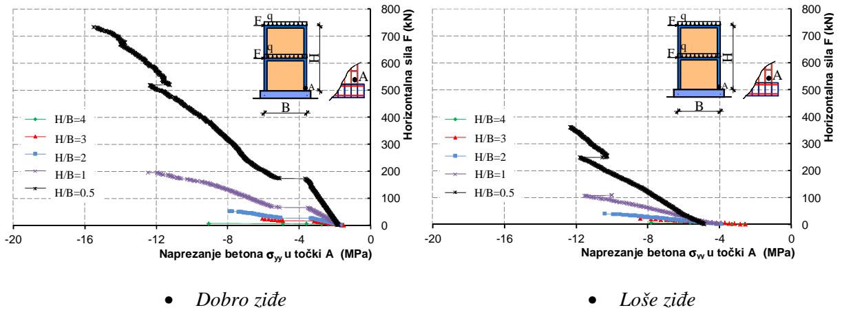
Slika 5.147. Vertikalno napreznja u betonu u točki A pri dnu omeđenih zidanih zidova
