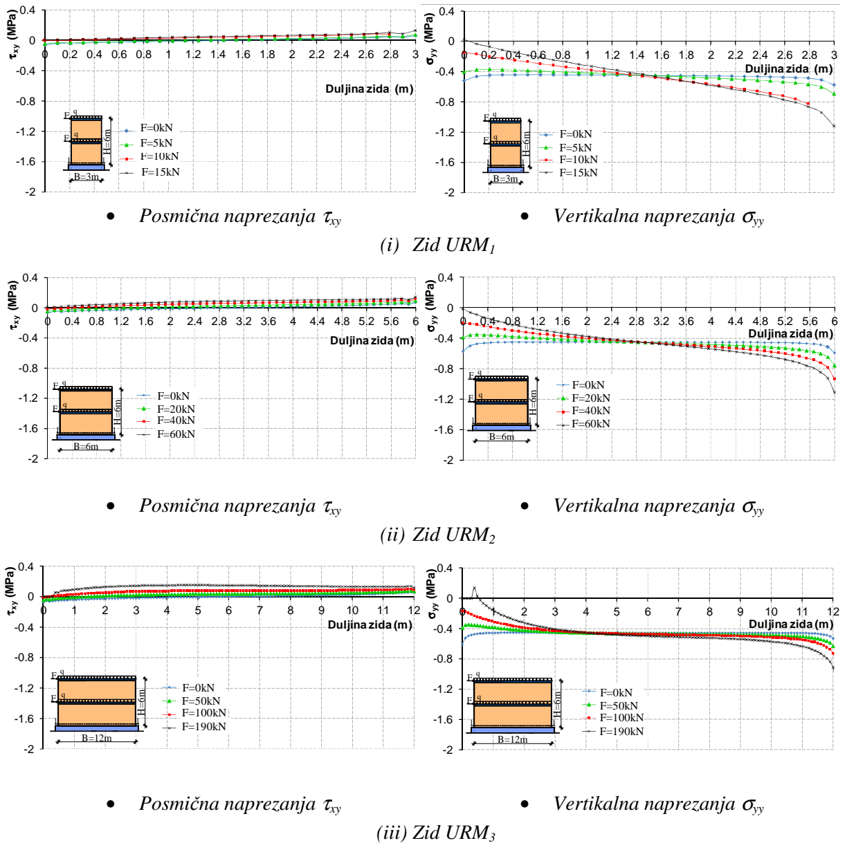
Slika 5.185. Prikaz napreznja u zidu pri temelju nearmiranih zidanih zidova s dobrim zidom za Model 1
