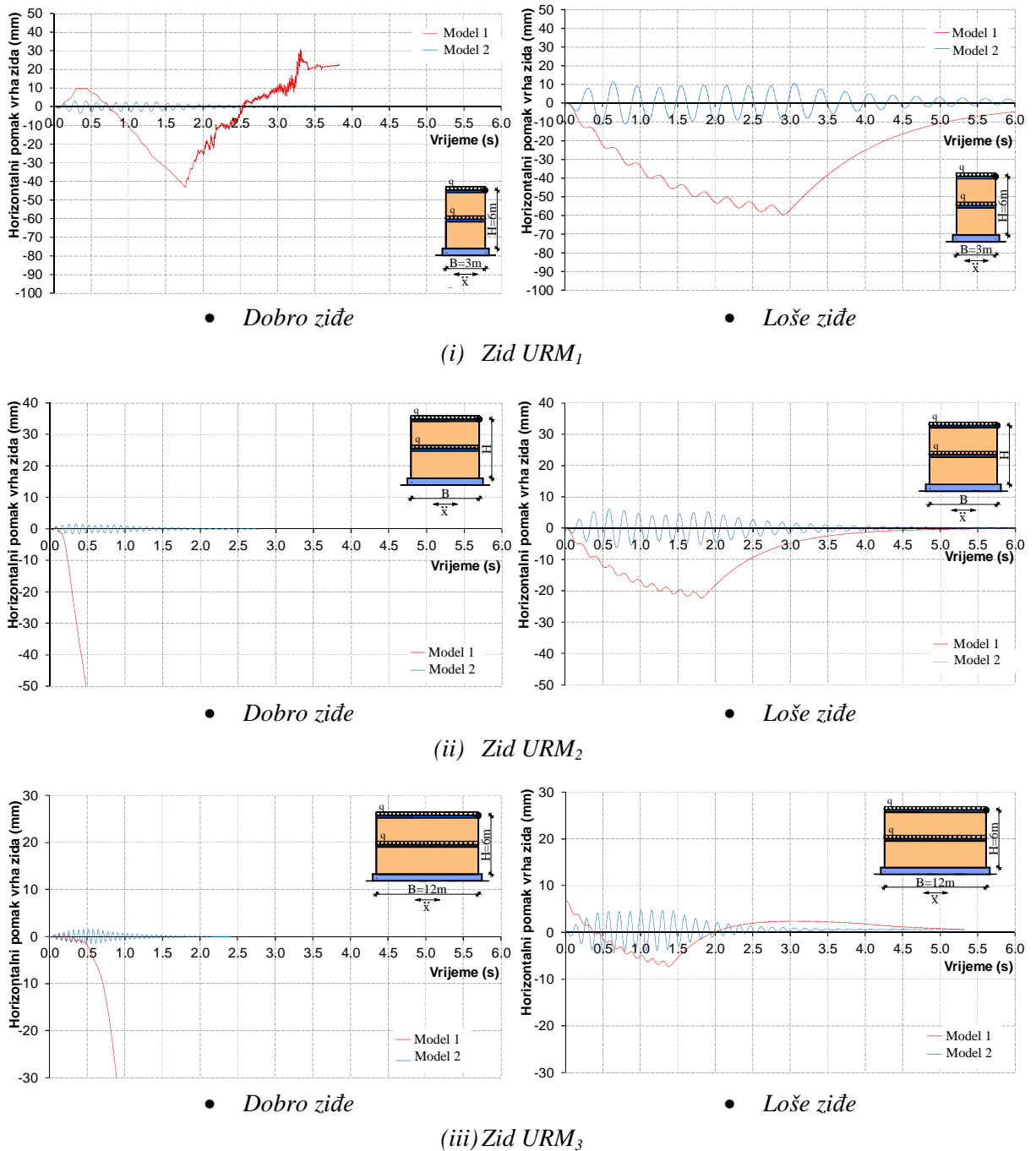
Slika 5.195. Horizontalni pomak vrha nearmiranih zidanih zidova izloženih harmonijskom ubrzanju podloge s a_{\max}=0,1g
