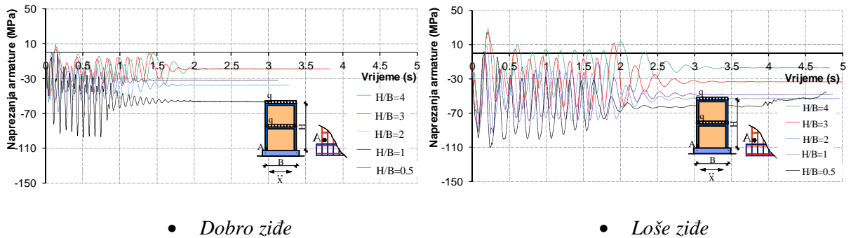
Slika 5.153. Naprezanje vertikalne armature u točki A pri dnu vertikalnih serklaža omeđenih zidanih zidova
