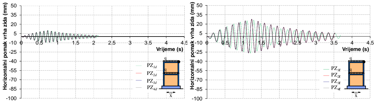
• Linearno-elastični model
