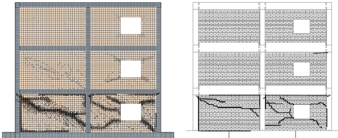
(i) Stanje pukotina - numerički model prikazan u Poglavljju 2
