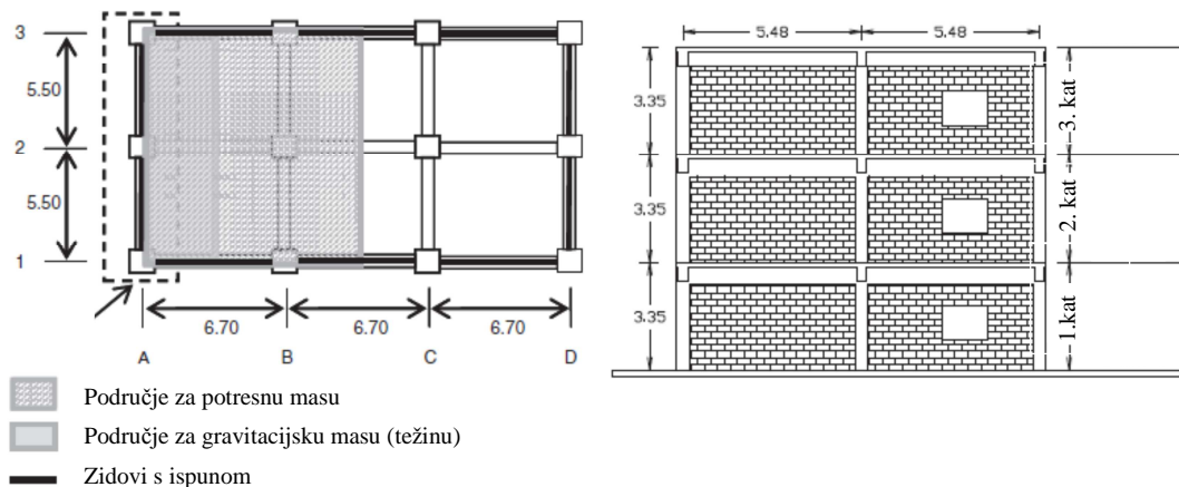
Slika 4.16. Prototip zgrade [321-323]
