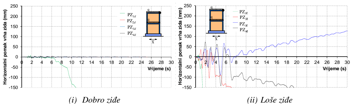
Slika 5.49. Horizontalni pomak vrha zidnih zidova bez otvora
