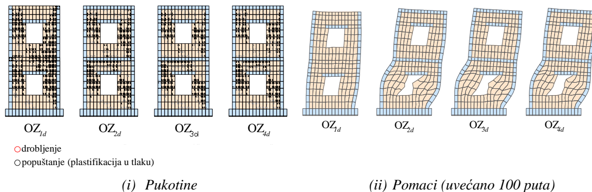
(i) Pukotine (ii) Pomaci (uvećano 100 puta) Slika 5.123. Pomaci i pukotine u zidanim zidovima s otvorima neposredno pred slom (dobro ziđe)
