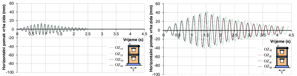
• Linearno-elastični model
