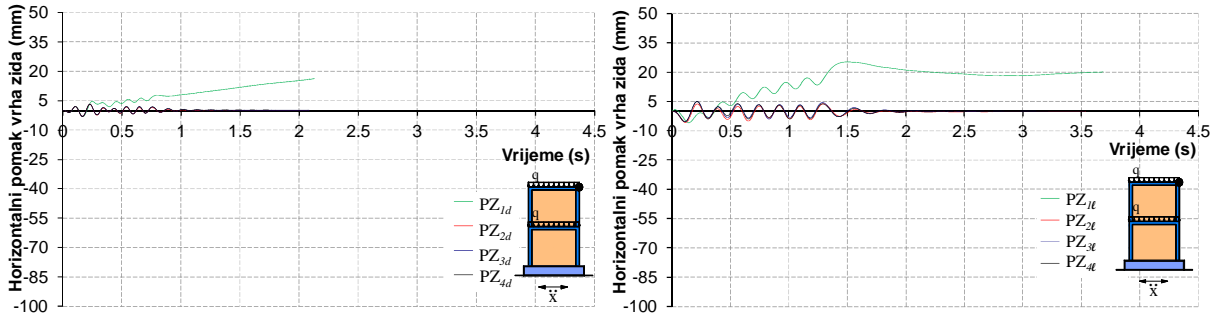
• Nelinearni model
