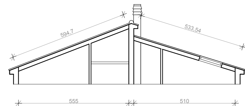
PRESJEK 2-2
