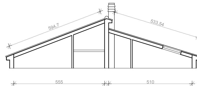
PRESJEK 2-2
