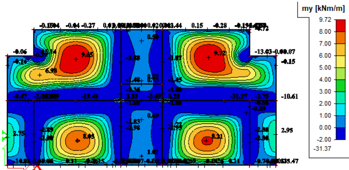
Slika 8.4 Moment savijanja (polje) M_{Ed,y} (kNm/m) za GSN-1
