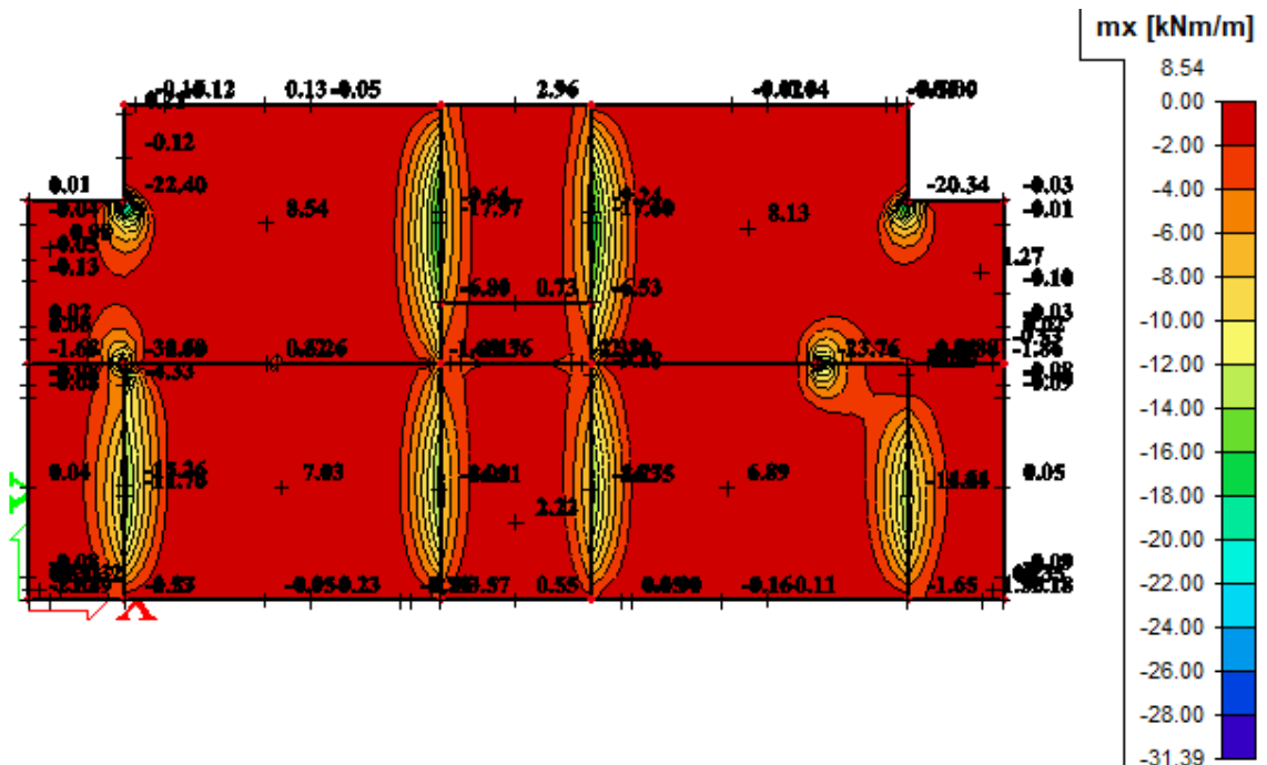
Slika 8.3 Moment savijanja (ležaj) M_{Ed,x} (kNm/m) za GSN-1
