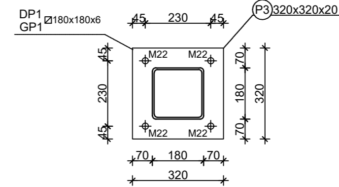
Presjek 4-4
