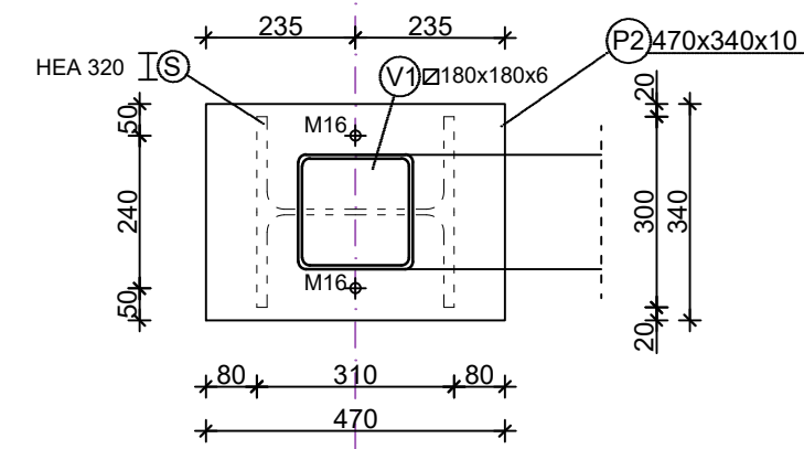
Presjek 2-2
