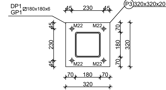
Presjek 4-4
