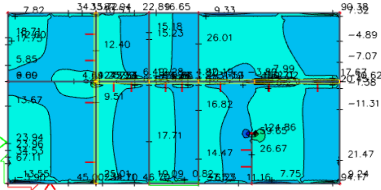
Slika 7.7 Poprečne sile V_{Ed,x} (kN/m) za GSN-1
