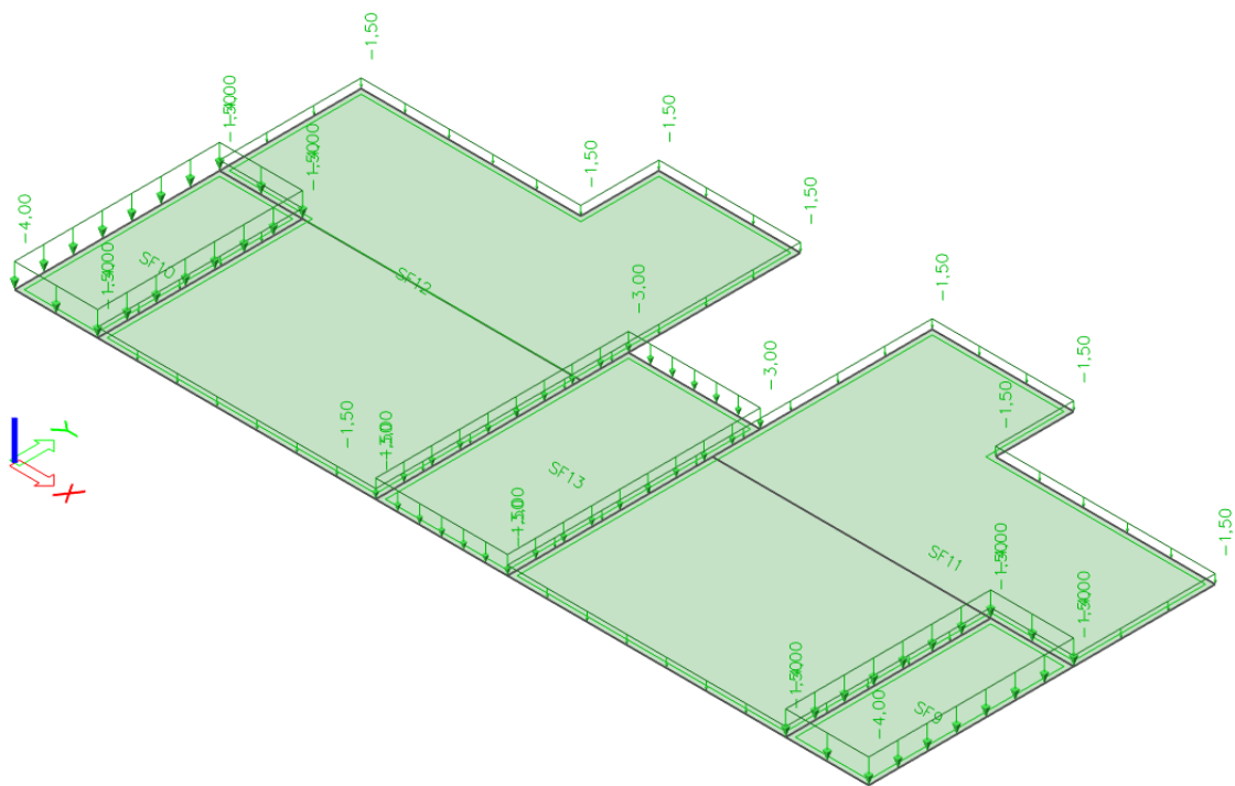
Slika 4.2 Promjenjivo djelovanje Q(\text{kN/m}^2)
