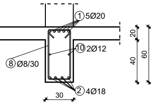
Presjek 1-1 (M 1:25)
