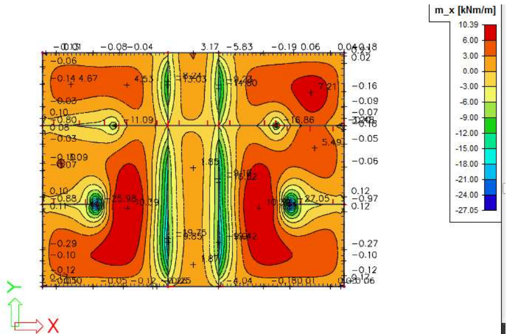
Slika 7.2 Moment savijanja M_{Ed,x} (kNm/m) za GSN-1
