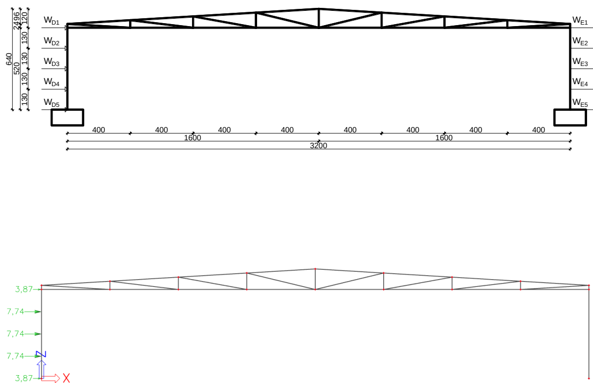
Slika 18. Raspodjela opterećenja vjetrom W_2 po čvorovima
