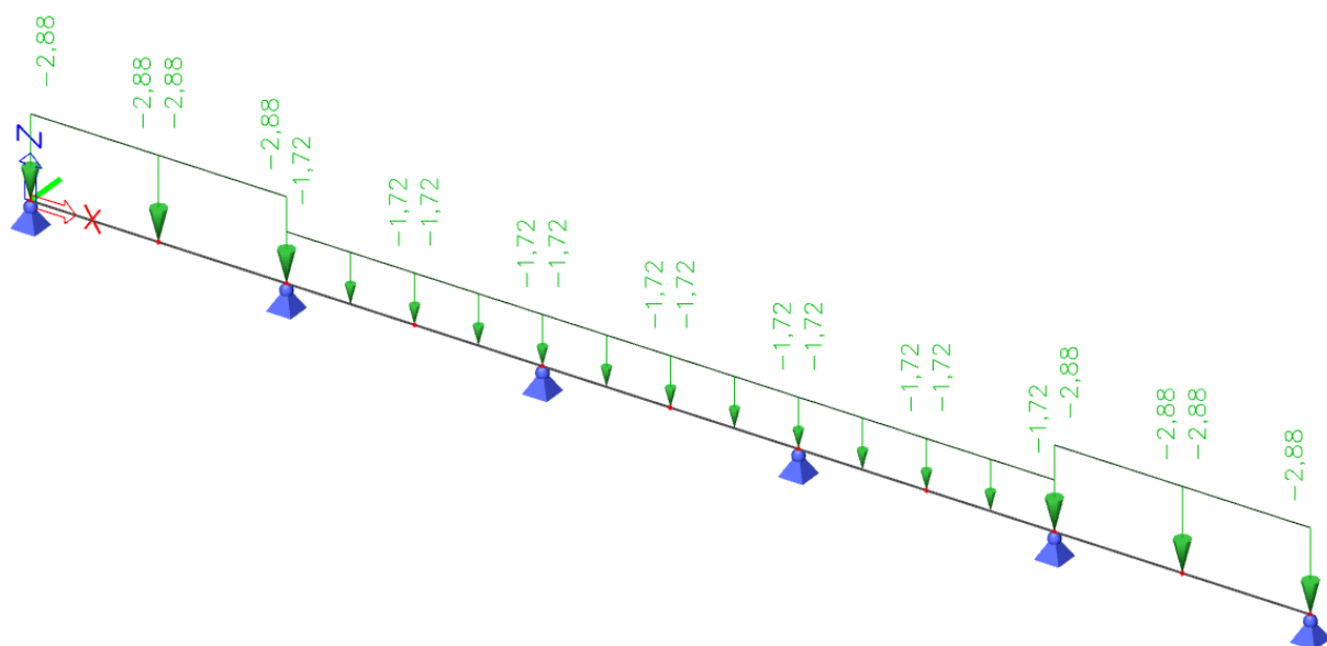
Slika 44. Raspodjela opterećenja vjetrom W_4
