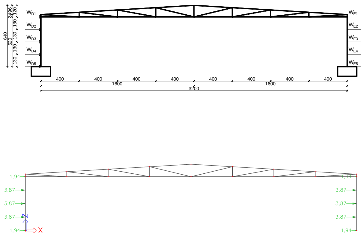
Slika 17. Raspodjela opterećenja vjetrom W_1 po čvorovima
