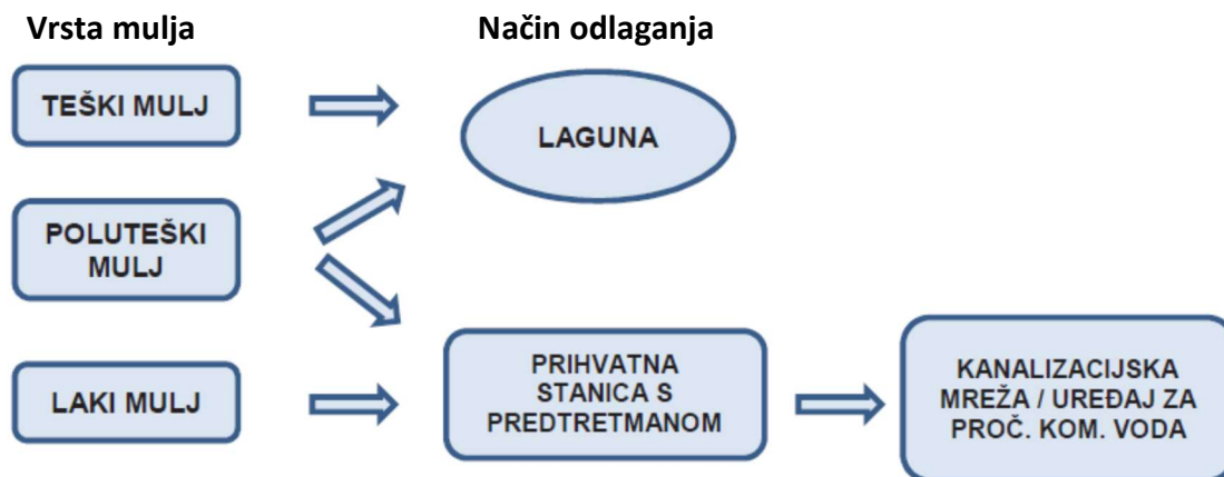
Slika 6.5. Shema privremenog rješenja odlaganja mulja
