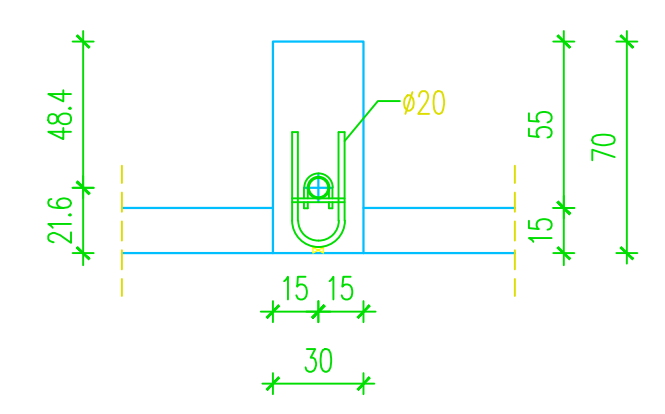
PRESJEK 3 – prijedlog rješenja držača nosača
