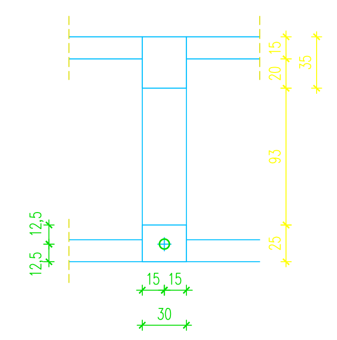
PRESJEK 10 – položaj kabela na sredini nosača
