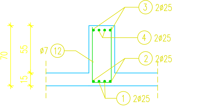
PRESJEK 5-5
