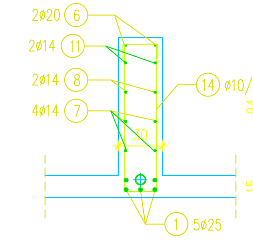
PRESJEK 2-2
