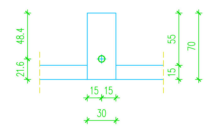
PRESJEK 3 – položaj kabela na čelo nosača
