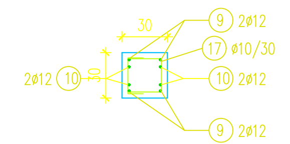
PRESJEK 4-4
