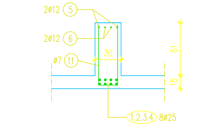
PRESJEK 4-4
