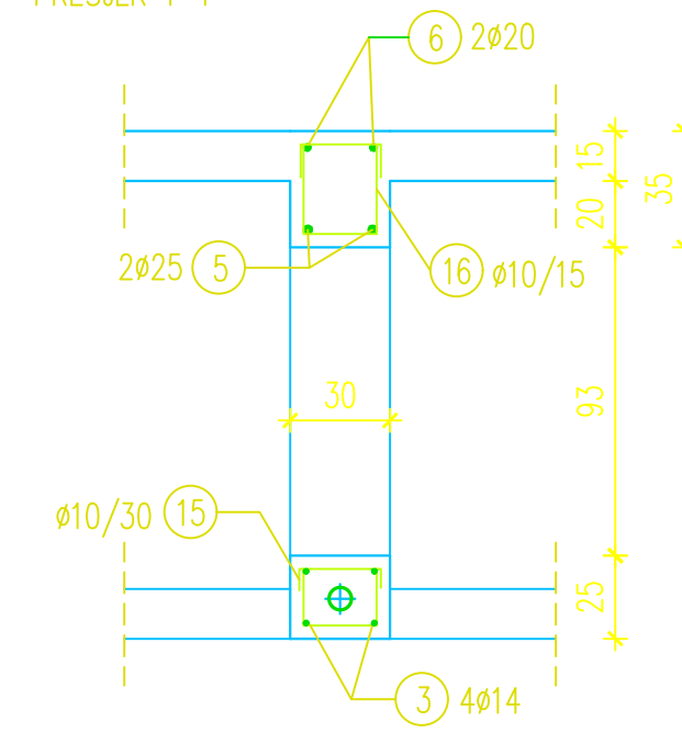
M=1:25 PRESJEK 1-1
