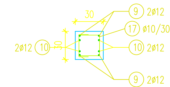
PRESJEK 4-4
