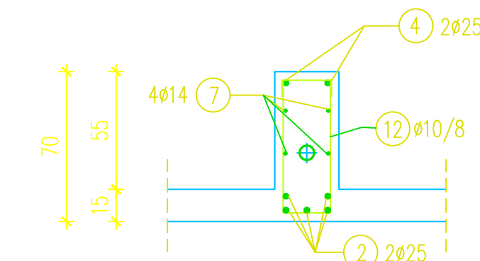
PRESJEK 3-3
