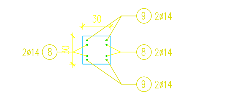
PRESJEK 6-6
