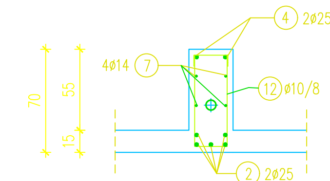
PRESJEK 3-3
