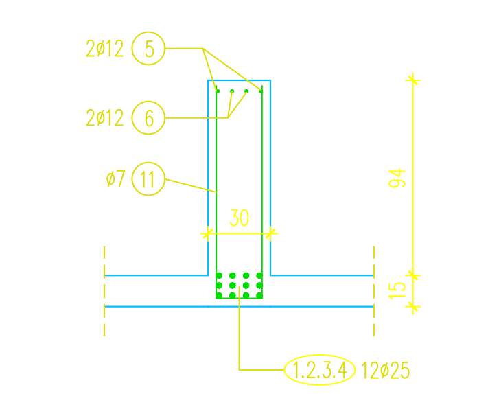
PRESJEK 3-3
