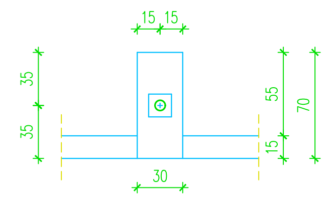
PRESJEK 0 – položaj kabela na čelo nosača
