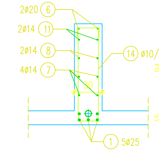
PRESJEK 2-2
