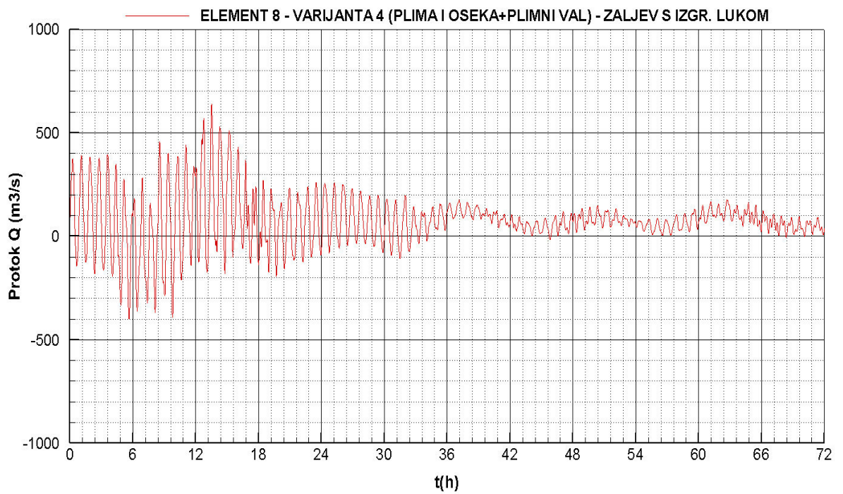
Slika 4.59 Protok – element 8
