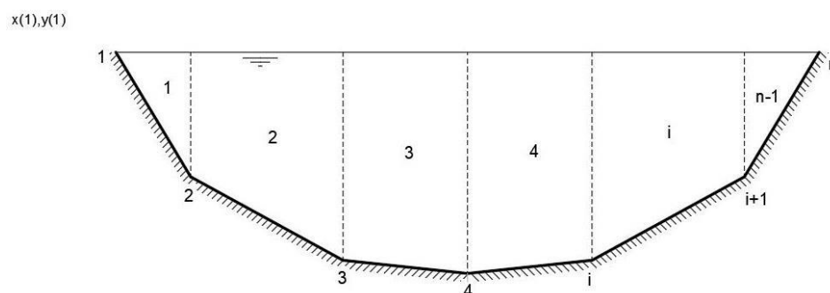
Slika 4.1 Shema poprečnog presjeka
