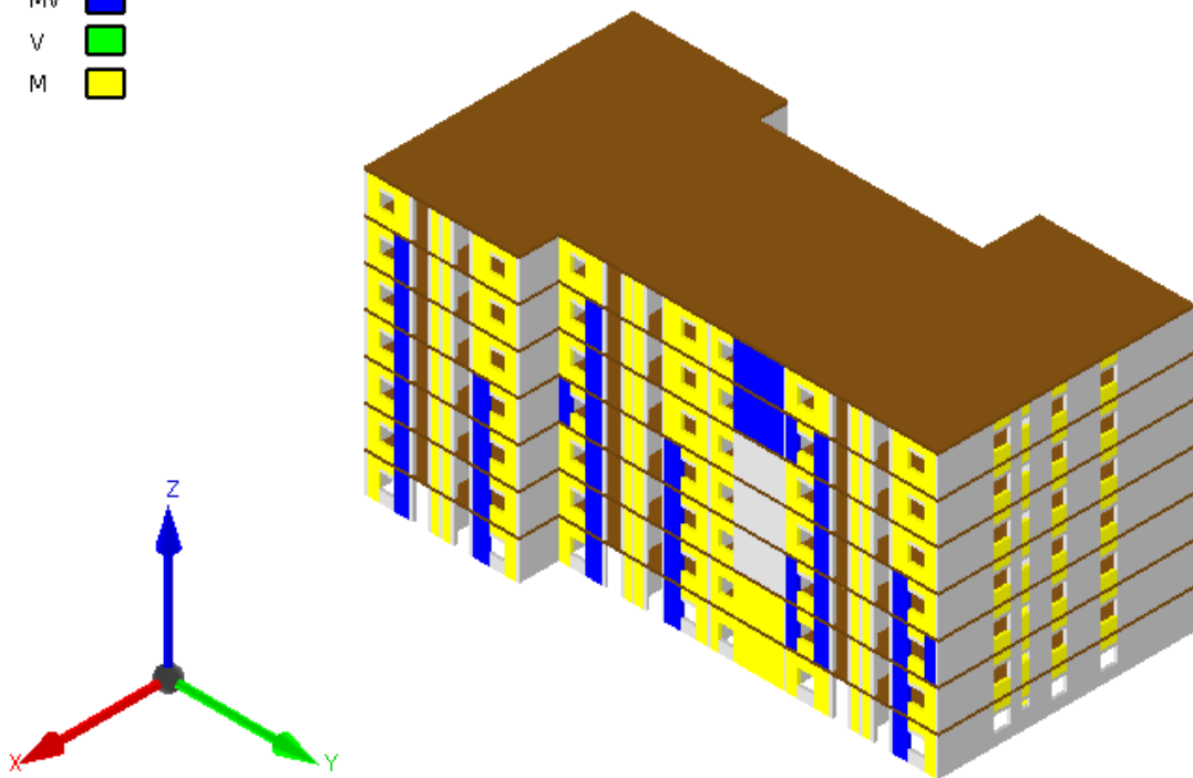
Slika 21 Oštećenje konstrukcije od ukupne slomne sile u smjeru-x
